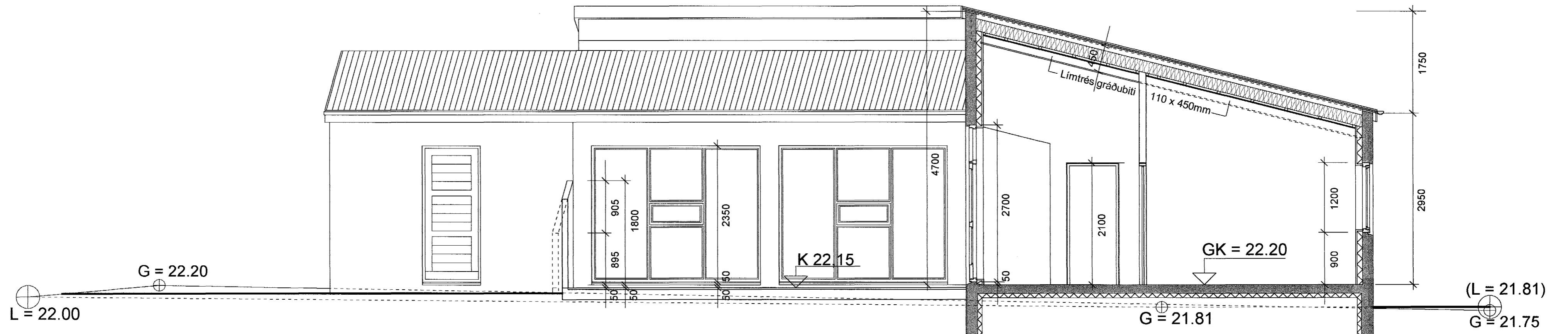
Sneiðing C - C
