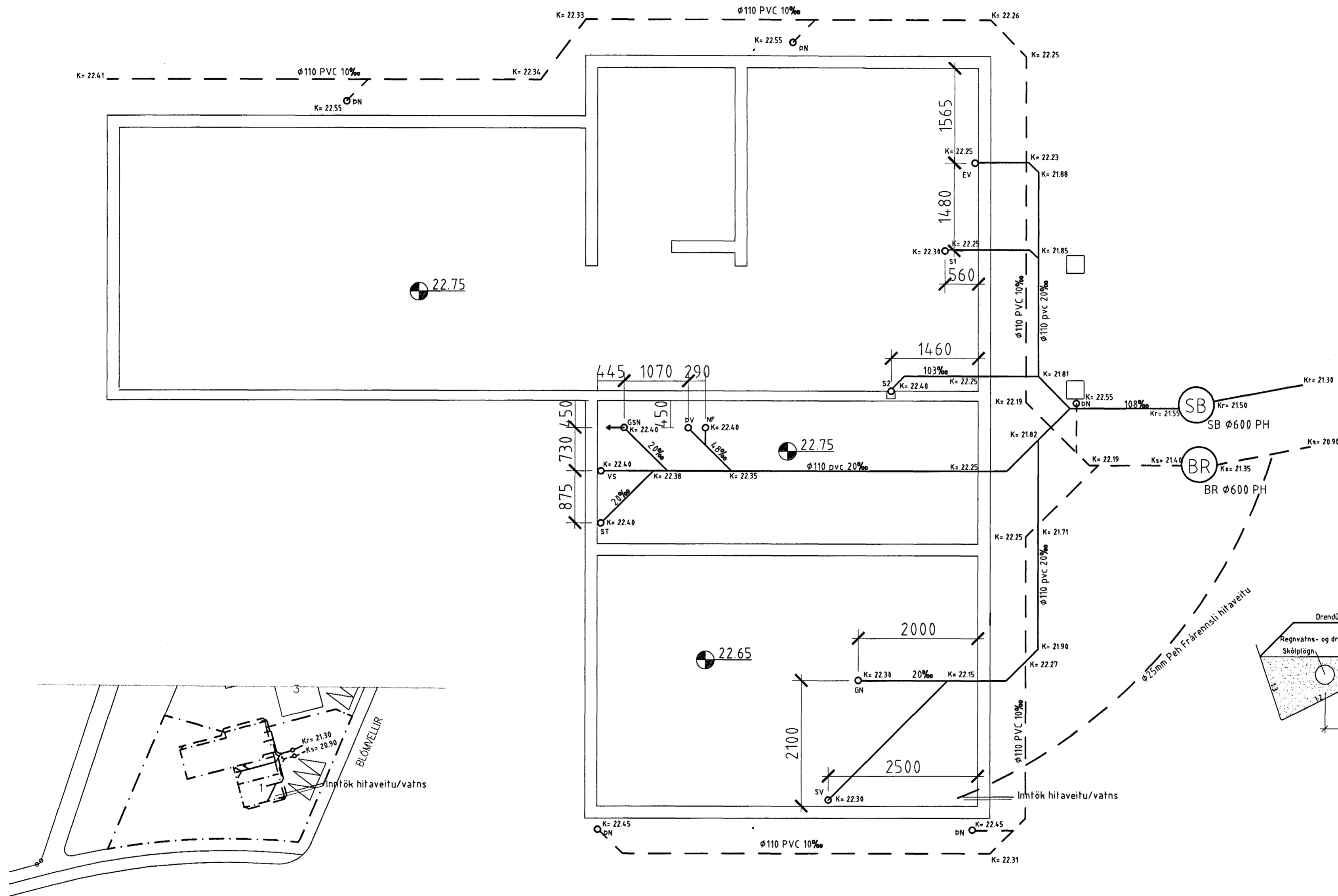
AFSTÖÐUMYND 1 : 500
