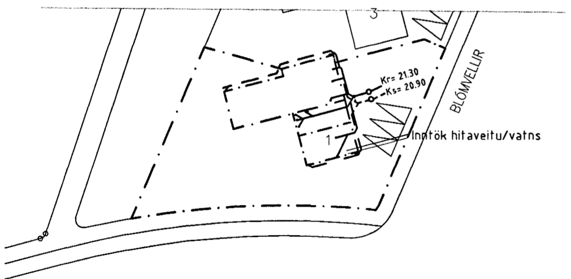
AFSTÖÐUMYND 1 : 500
