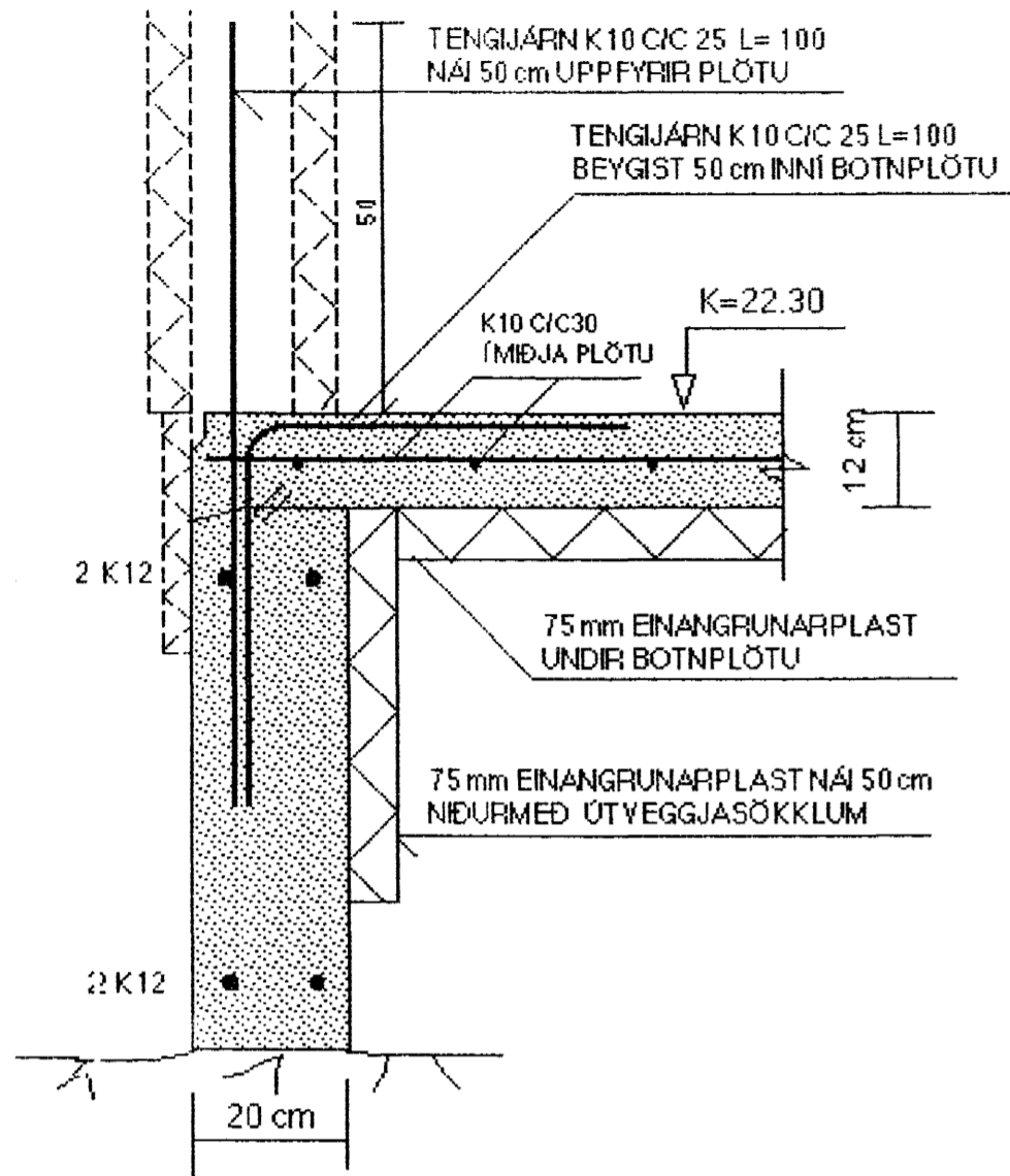
SNID D-D MKY. 1:10
