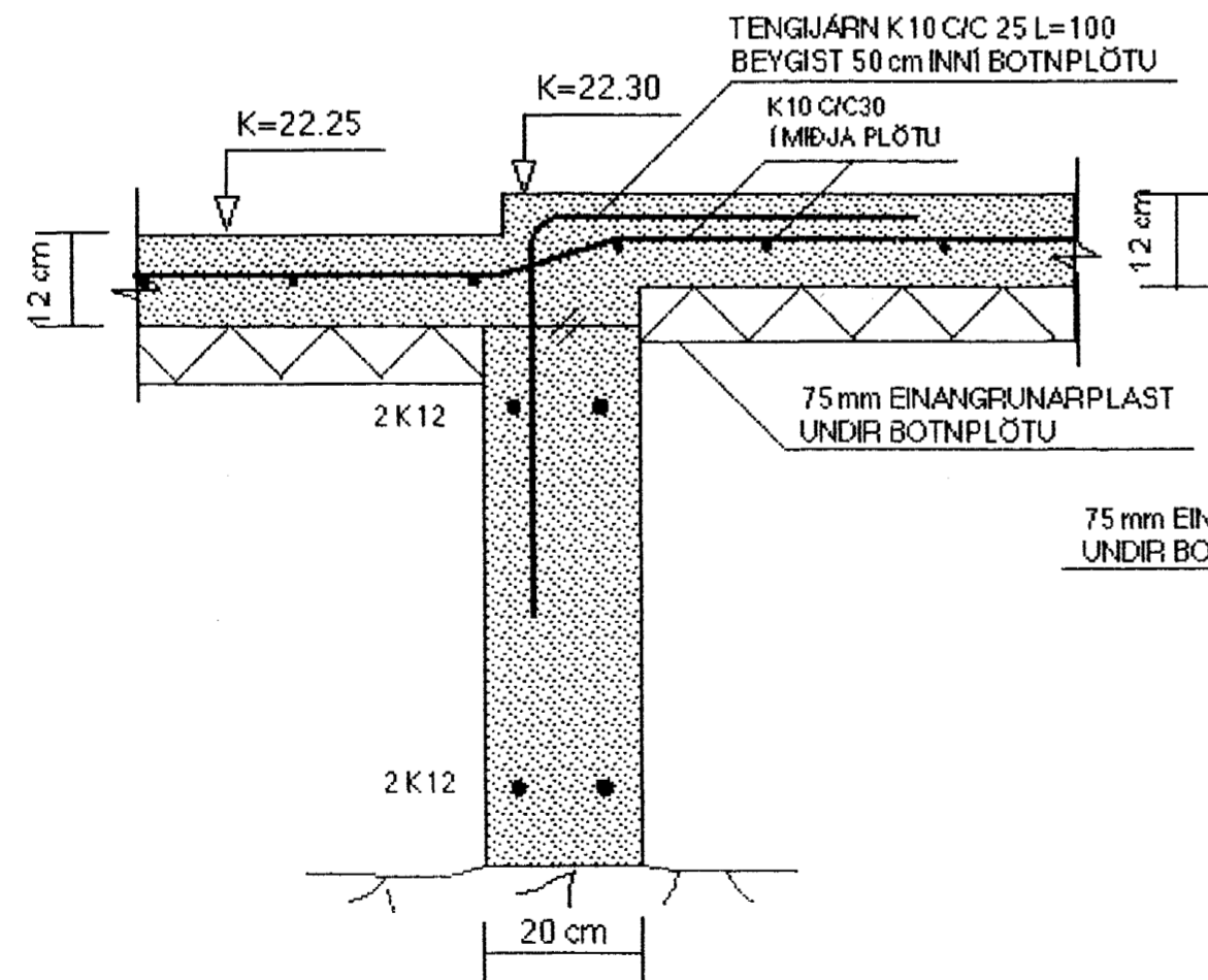
SNID D-D MKY. 1:10
