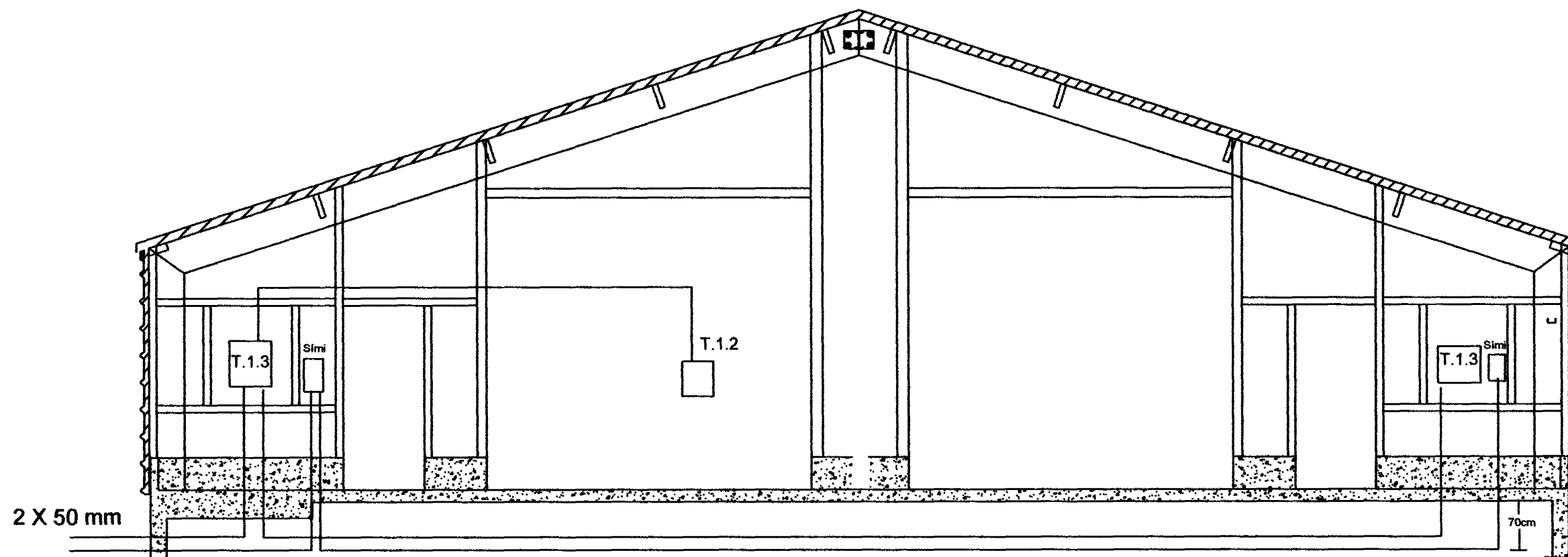
B 101 Snið A-A Mælikvarði 1:100
