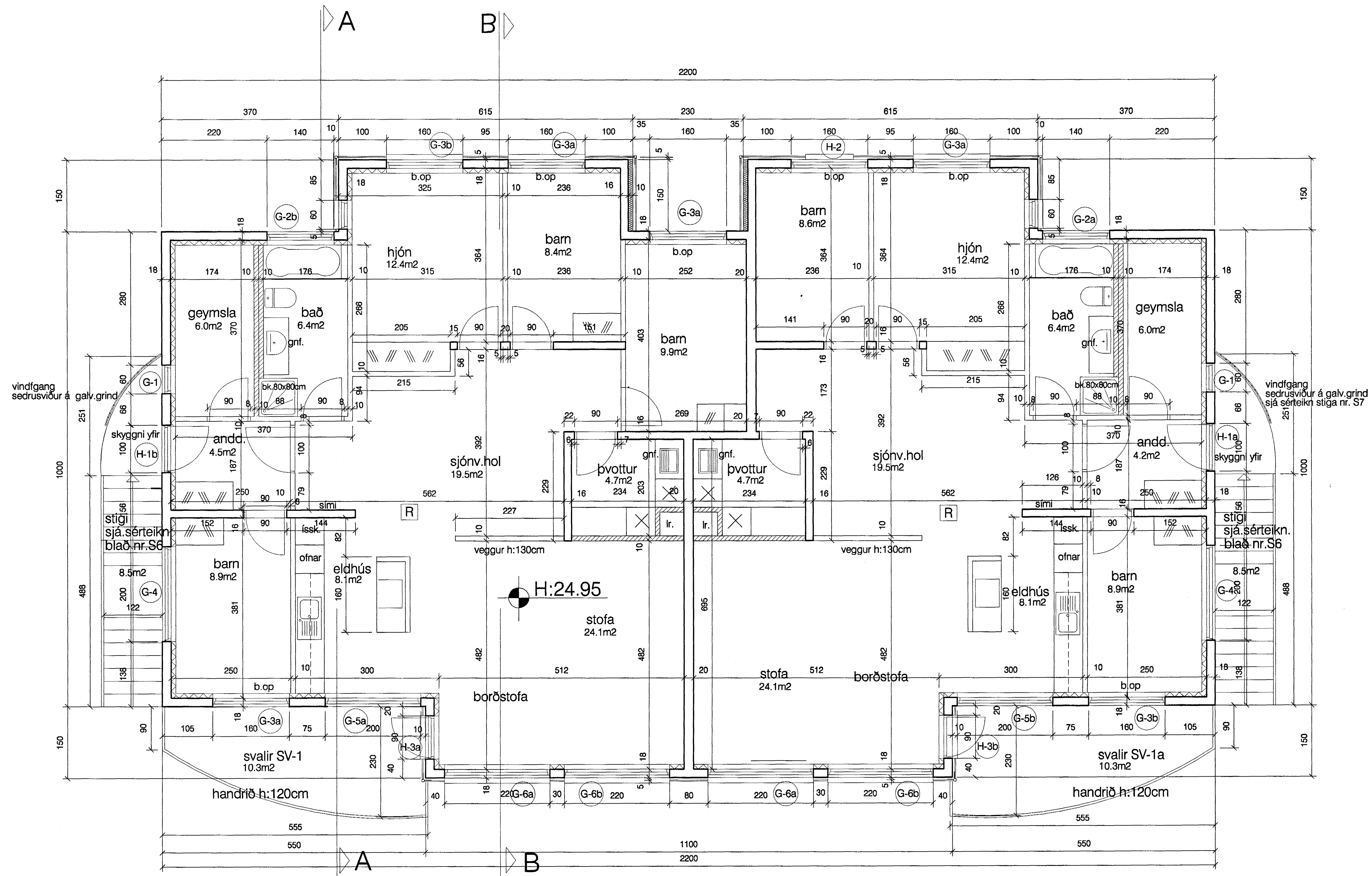
grunnmynd 2. hæð
