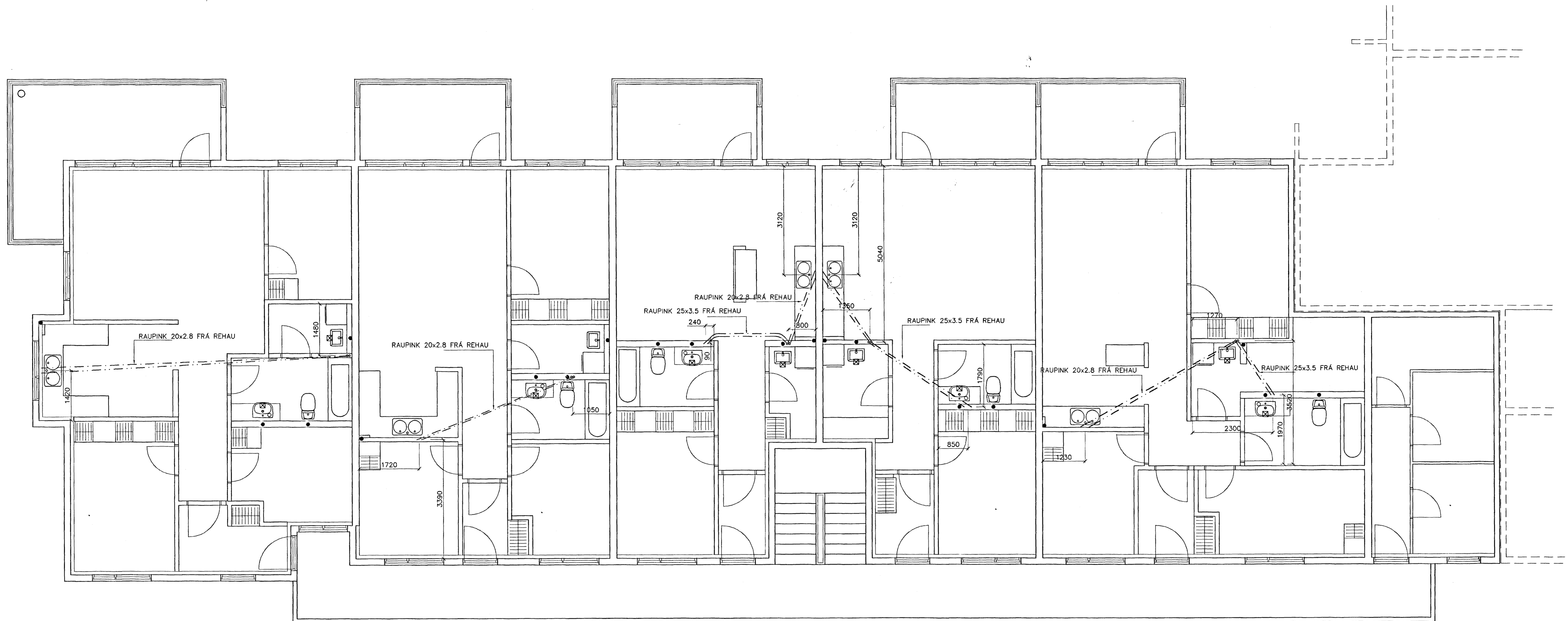
GRUNNMYND 2 HÆÐAR 1:50
