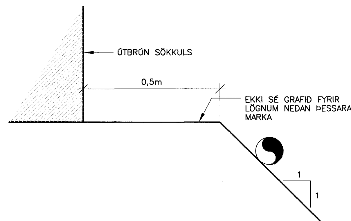
LEGA LAGNA VÍÐ HÚS 1:10
