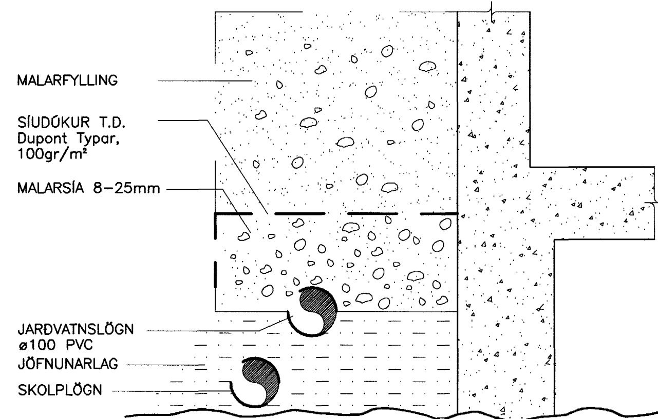
FRÁGANGUR JARDVATNSLAGNA ÓR PVC 1:10
