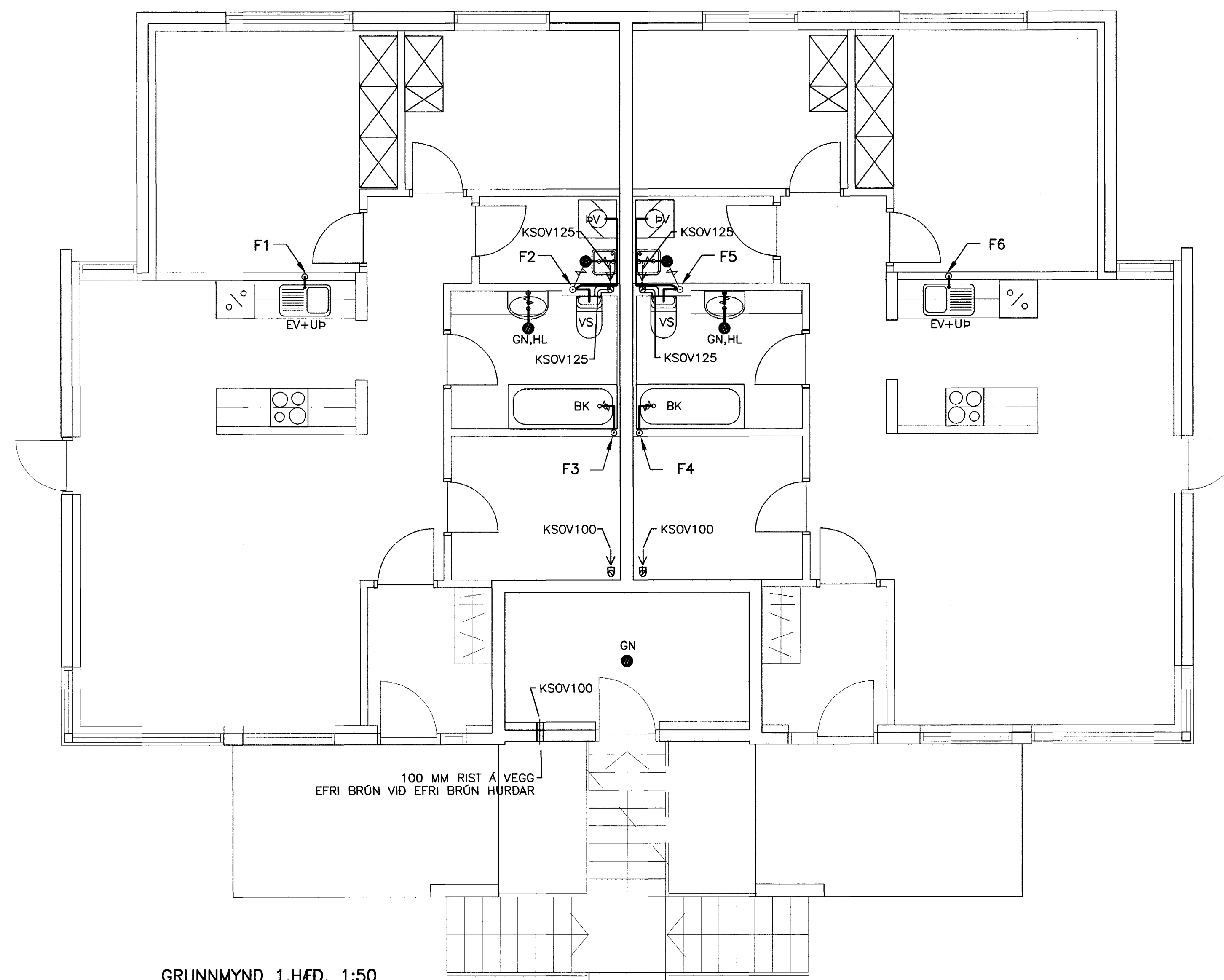
GRUNNMYND 1.HÆÐ, 1:50
