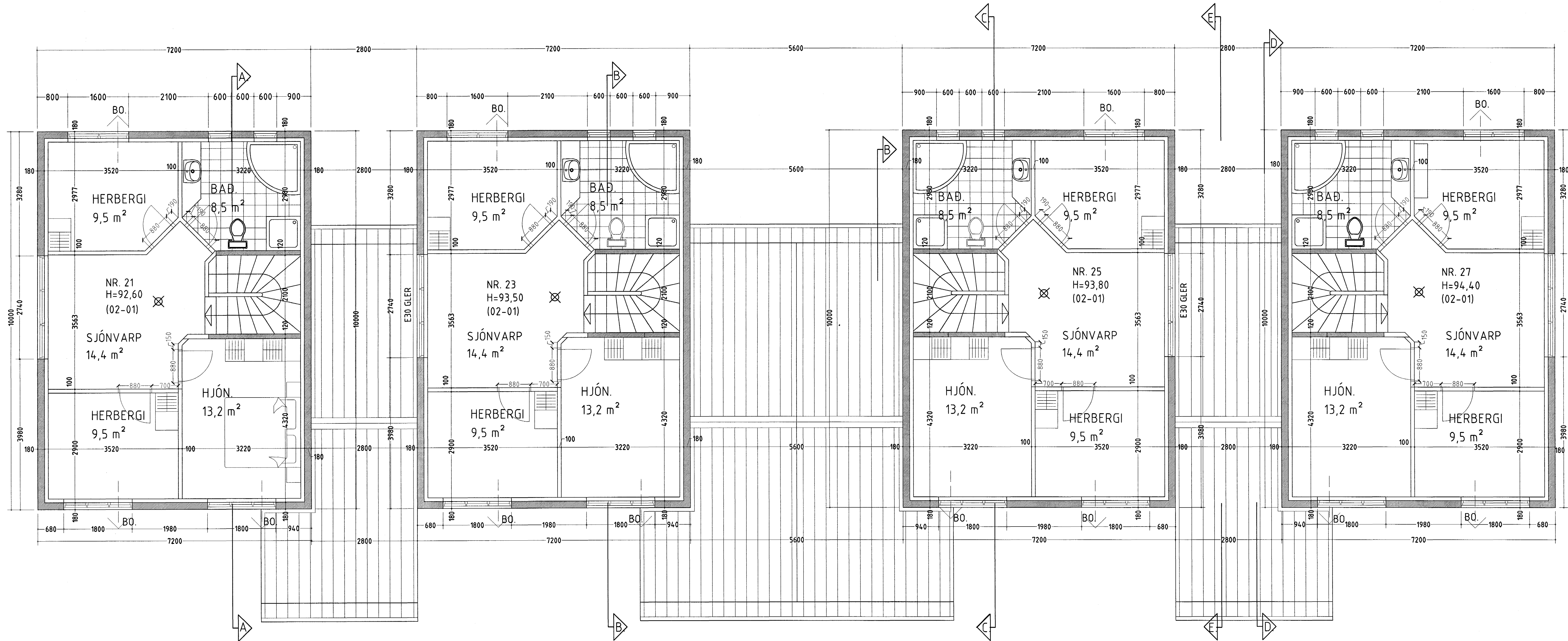
GRUNNMYND 2. HÆÐ. MKV. 1:50.
