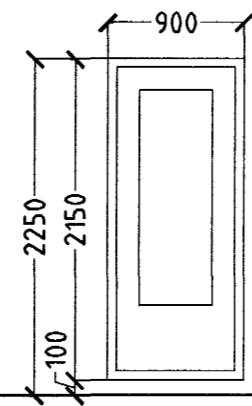
4 STK. STOFA. HURÐ OPNAST VINSTRI ÚT. 1 STK. STOFA. HURÐ OPNAST HÆGRI ÚT.
