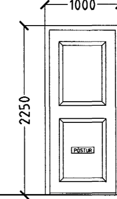
1 STK. ANDDYRI. ÍBÚÐ. 01-01. HURÐ OPNAST HÆGRI INN.
