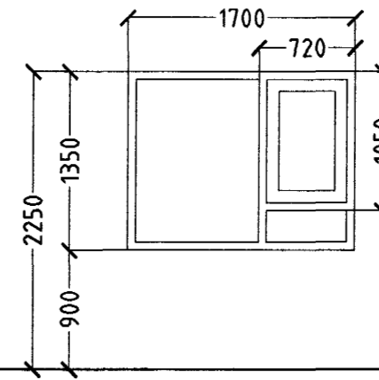
8 STK. HJÓN/HERB./ ELDHÚS. BJÖRGUNAROP.
