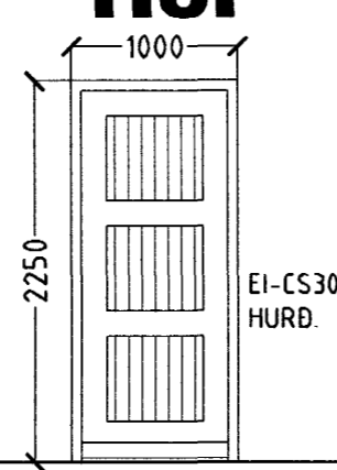
3 STK. STIGAHÚS. HURÐ OPNAST HÆGRI INN. 1 STK. STIGAHÚS. HURÐ OPNAST VINSTRI INN.
