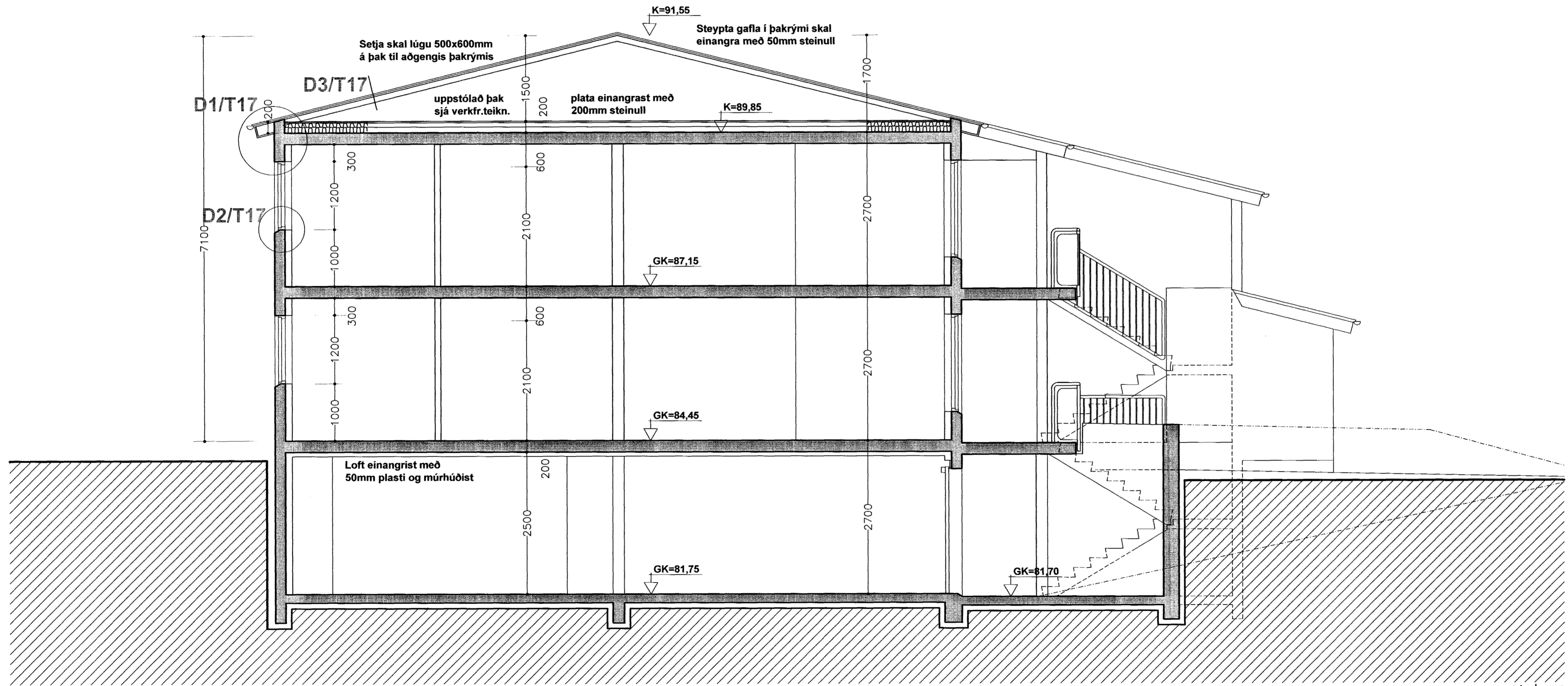
Snið A-A
