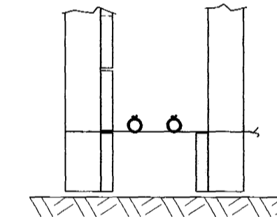
SNID C Í SÖKKULVEGG SÝND ERU 2 NEDSTU STEYPU- STYRKTARJARNIN Í STEYPUMÖTI OFAN Á NEDSTU MÖTAVIRUM.
