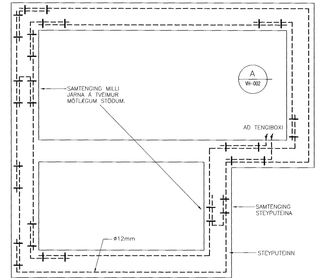
GRUNNMYND SÖKKULVEGGJA
