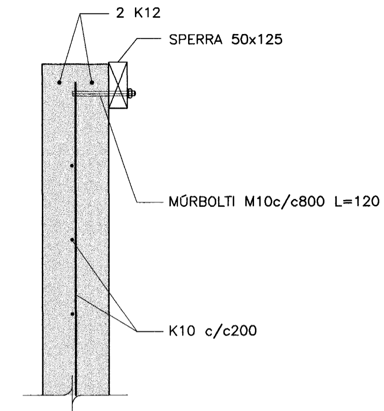
04 DEILI 231 1:10
