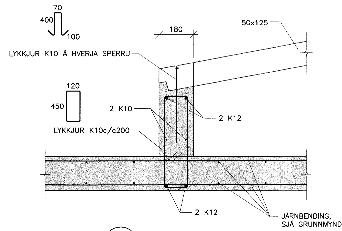
01 DEILI 231 1:10
