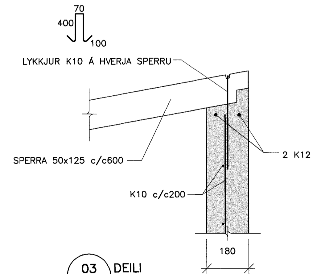
03 DEILI 231 1:10
