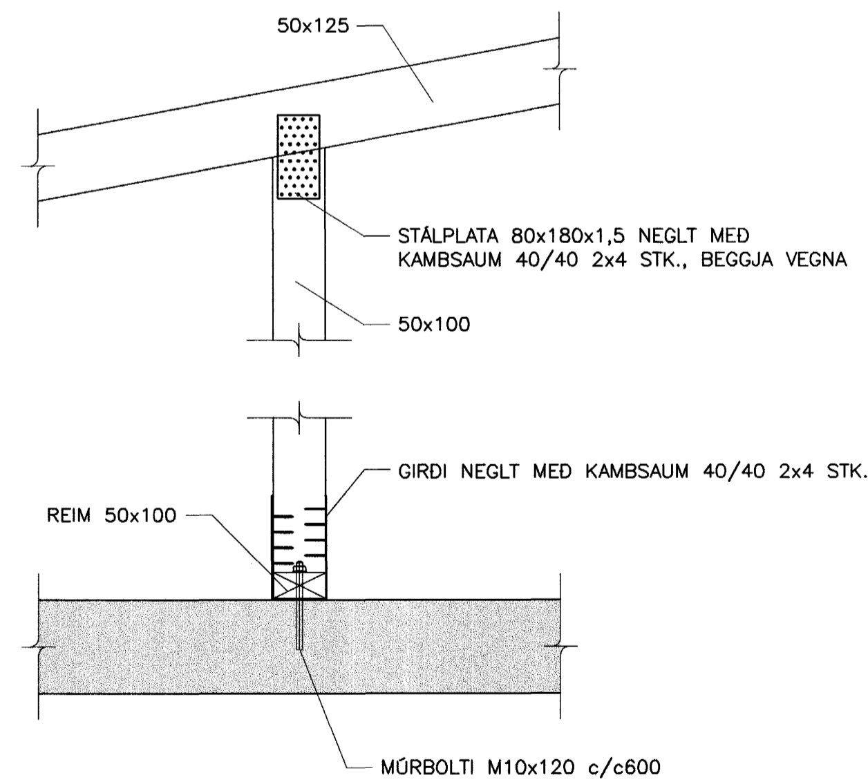
02 DEILI 231 1:10
