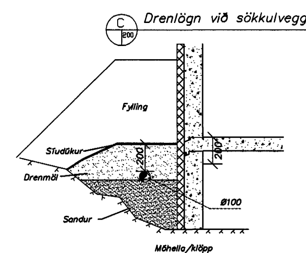
Frágangur á drenni (þerrilögn) við sökkulvegg
