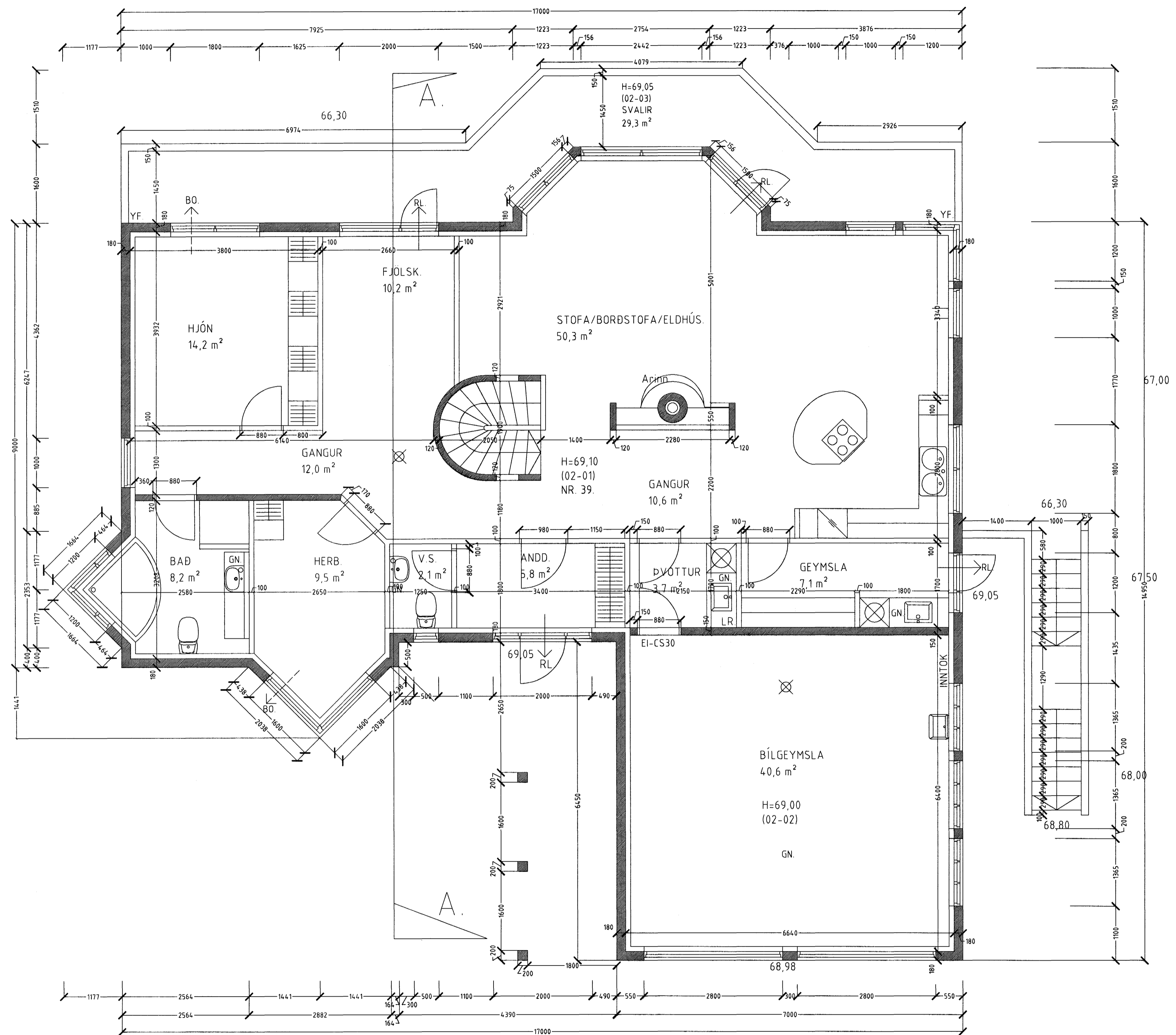
GRUNNMYND 2. HÆÐ MKV 1:50.
