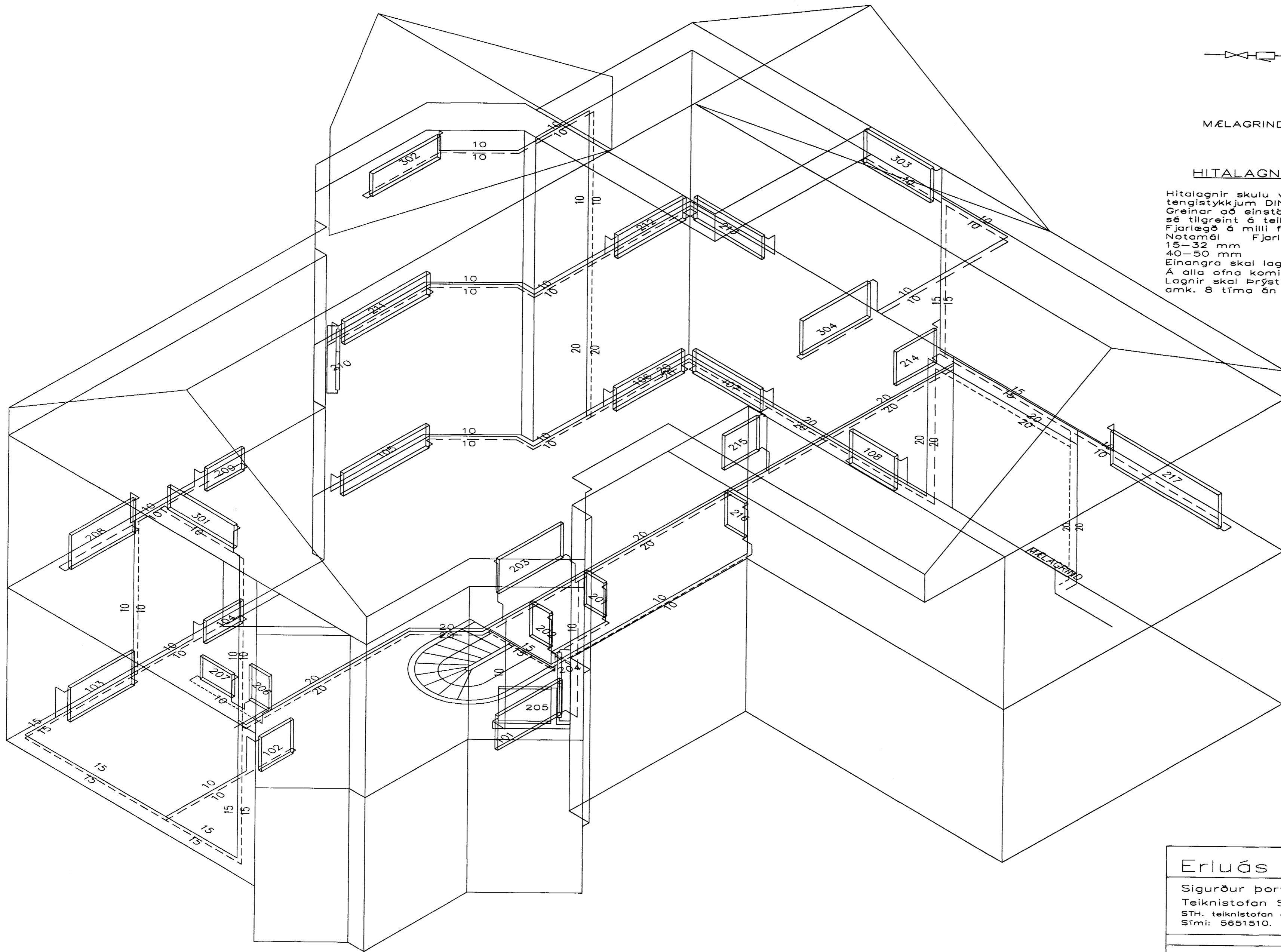
RÚMMYND HITALAGNA 1:50
