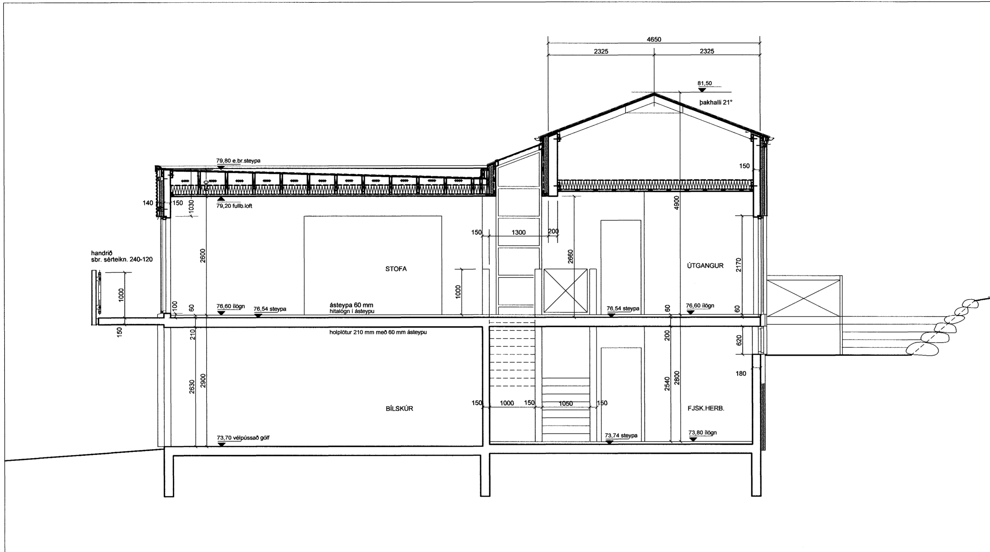
snið A - A, m = 1:50
