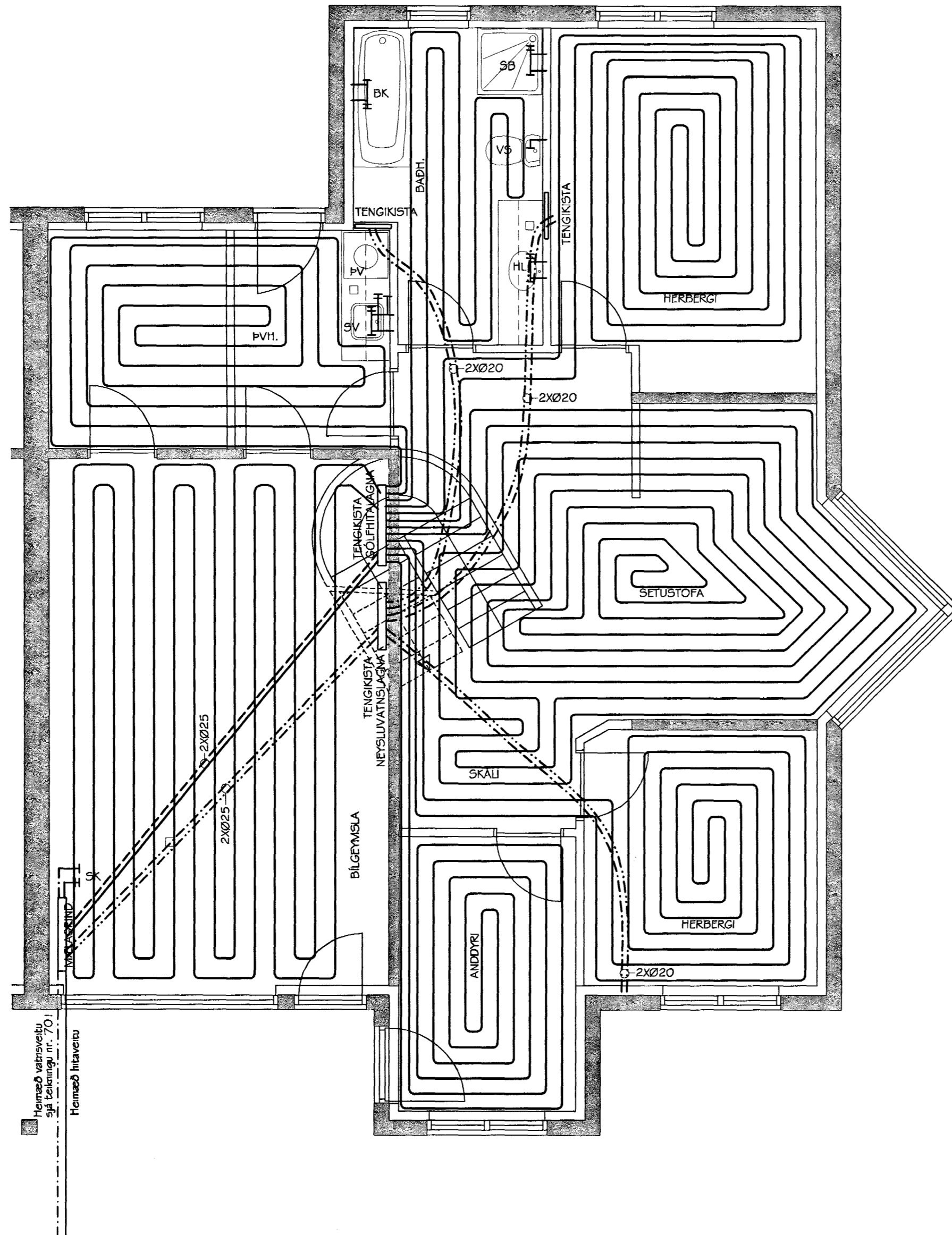
SVÖLUÁS 5 NEYSLUVATNS- OG HITALAGNIR GRUNNMYND NEDRI HÆÐAR MKV. 1:50
