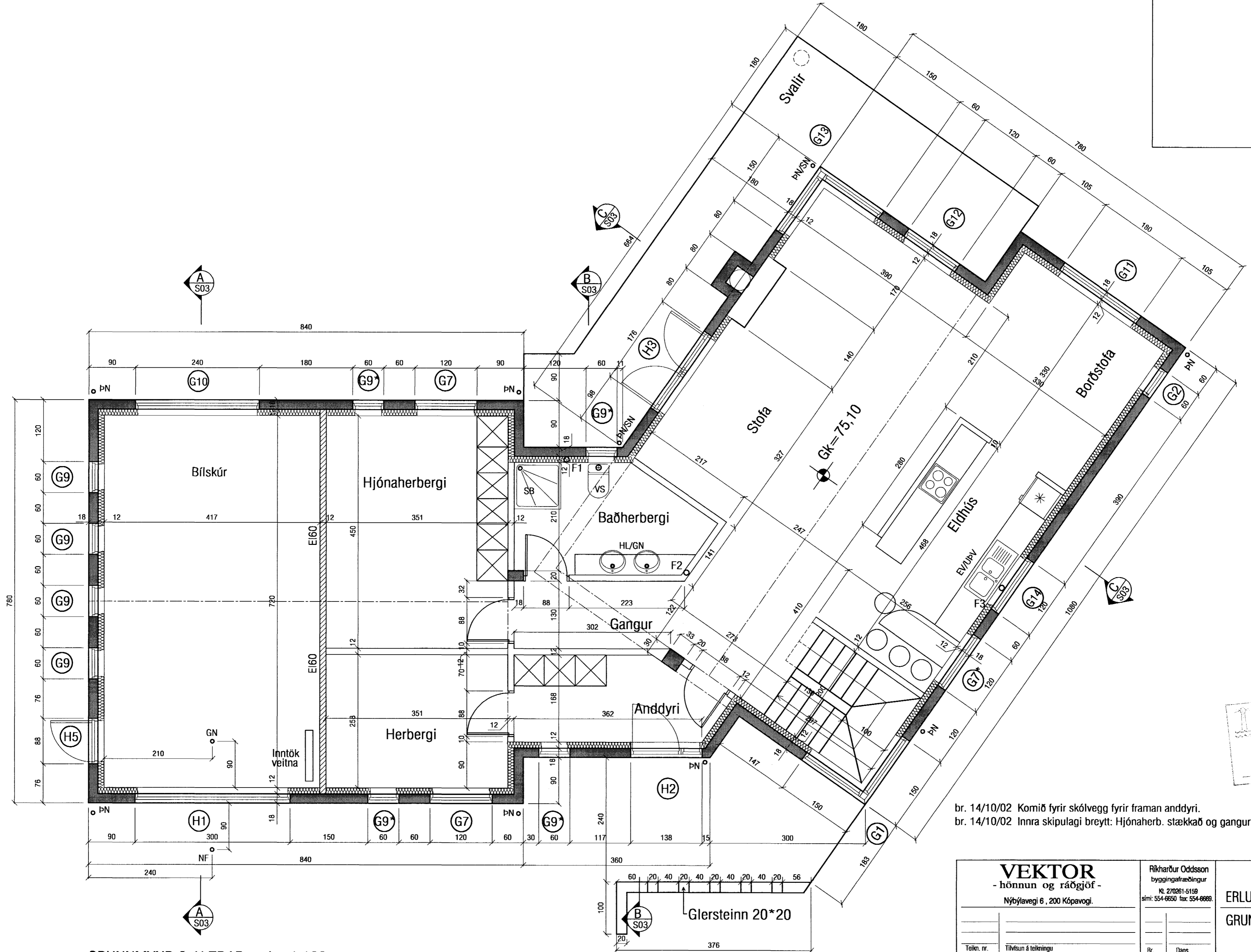
GRUNNMYND 2. HÆÐAR m.k.v 1:100
