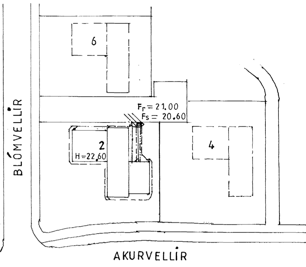
AFSTÖÐUMYND M ; 1:500
