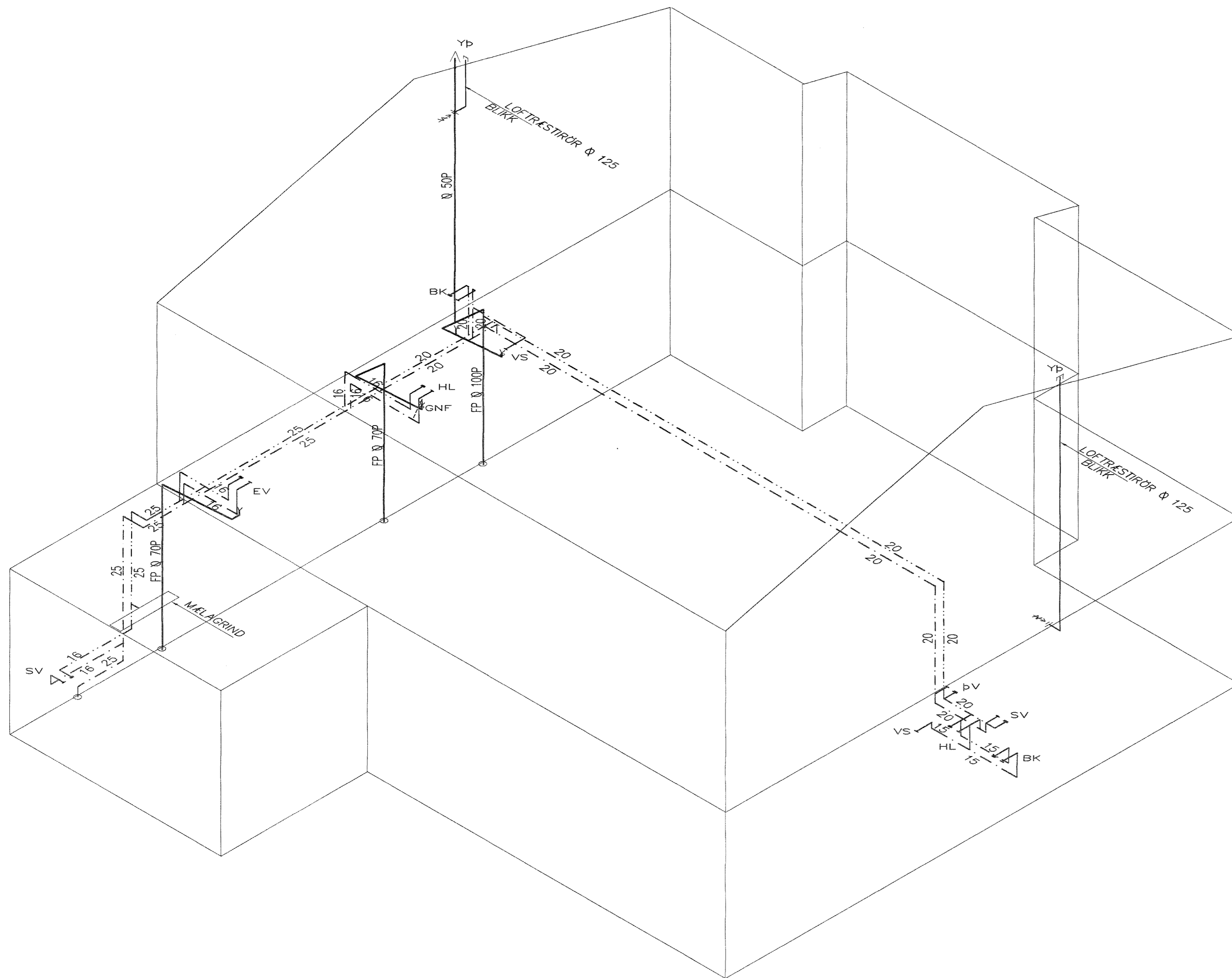
RÚMMYND VATNS OG FRÆRENNSLISLAGNA 1:50
