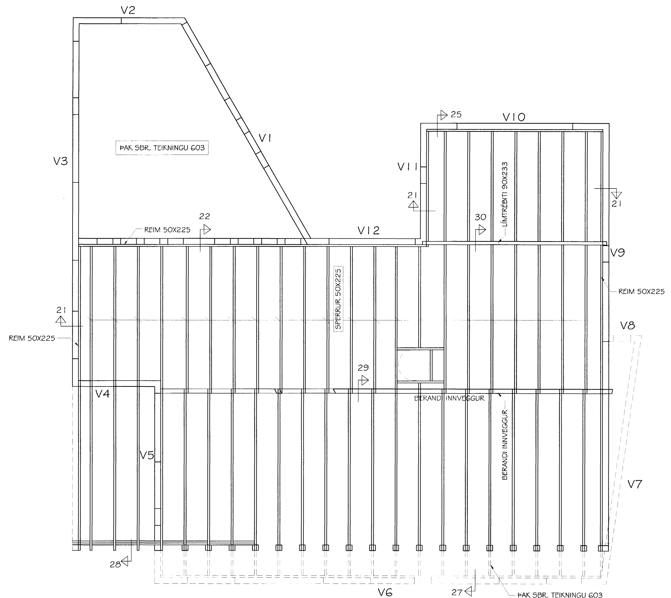
GRUNNMYND PÁKVIÐA - HALLANDI ÞÖK MKV. 1:50
