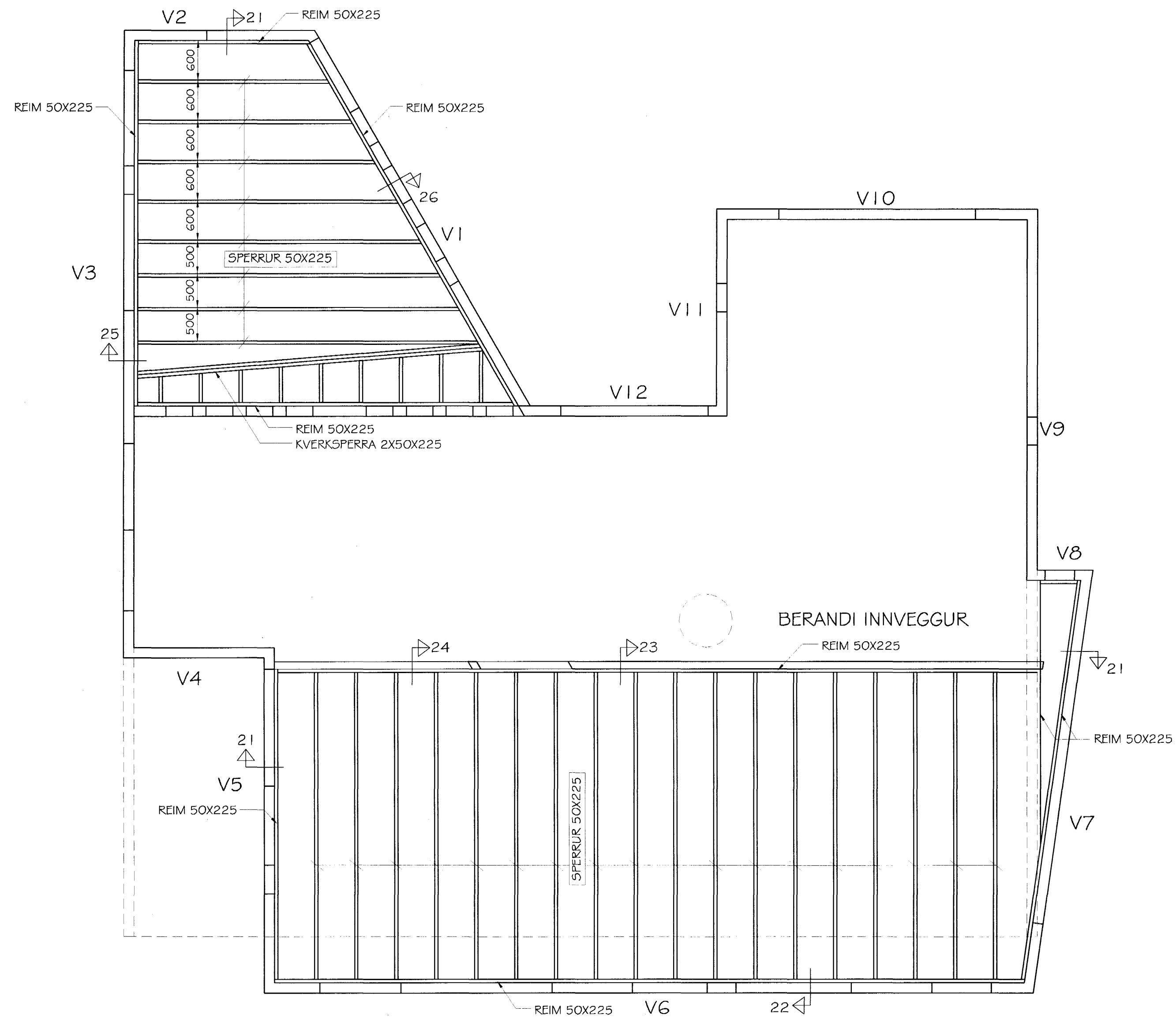
GRUNNMYND PÁKVIÐA - FLÖT ÞÖK MKV. 1:50
