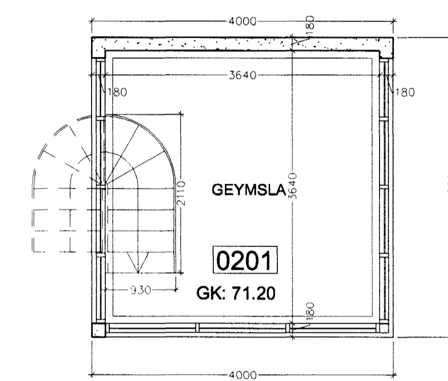
GRUNNMYND 2.HÆÐ
