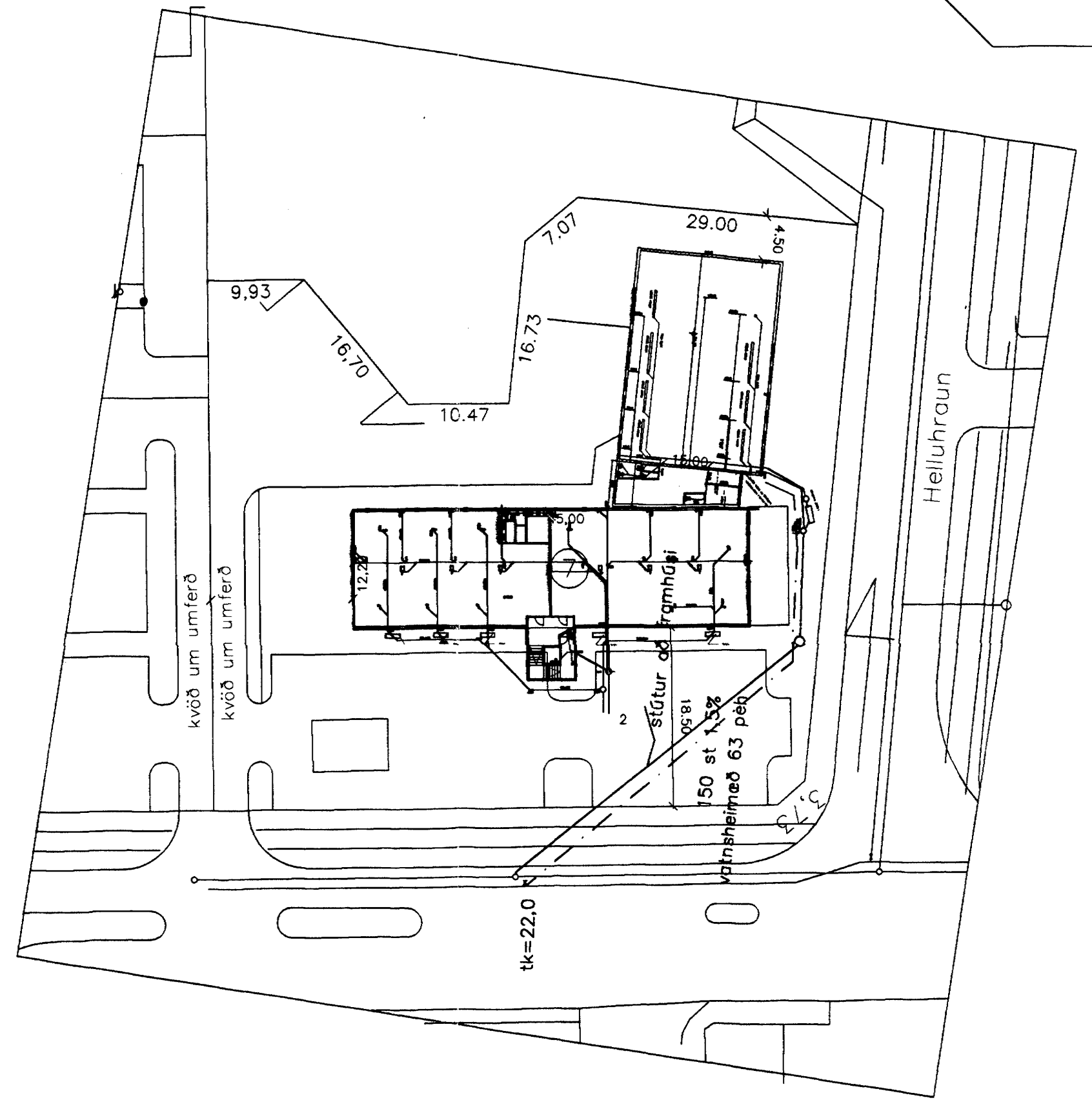
AFSTÖÐUMYND 1:500
