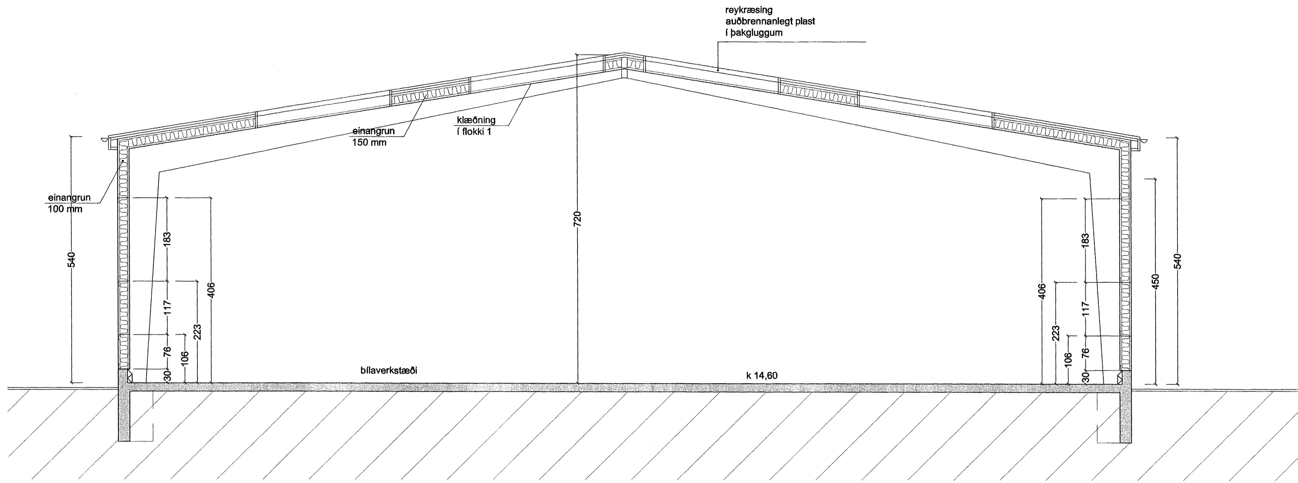
SNEIÐING A - A M 1:50
