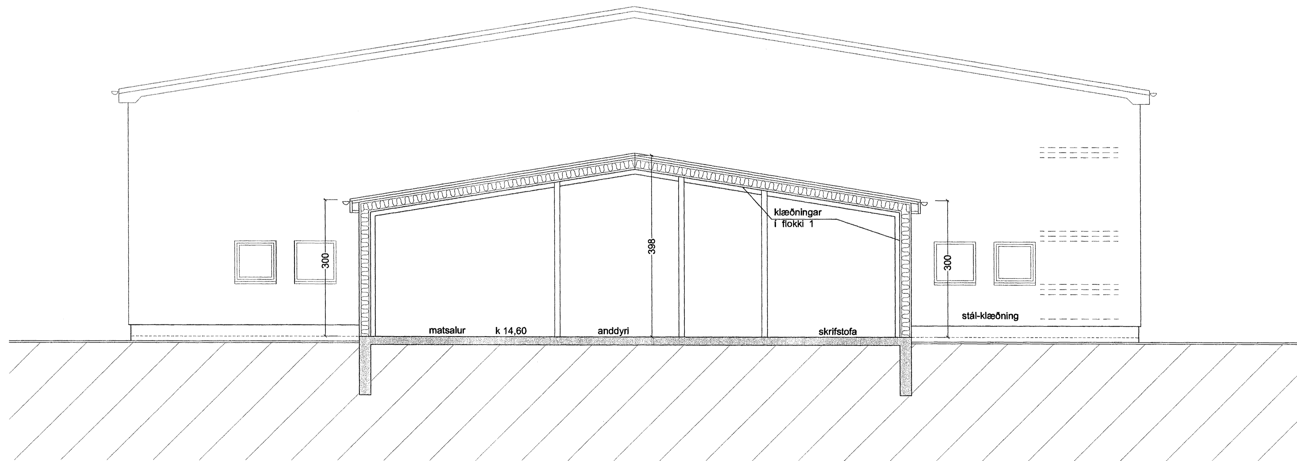
SNEIÐING B - B M 1:50
