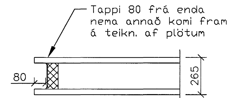
Snið í enda holplatna Mælikvarði 1:20
