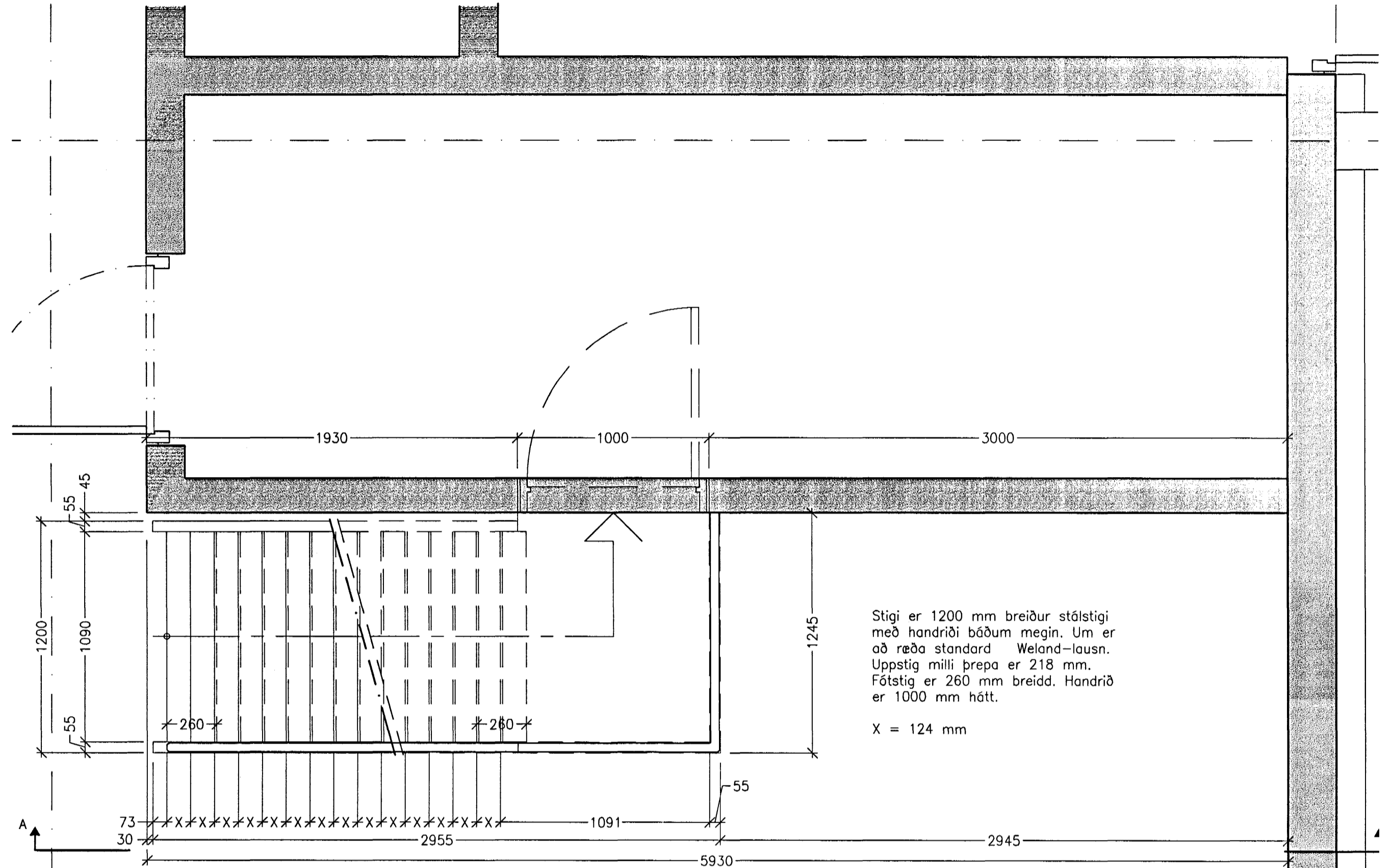
Grunnmynd stálstiga í tækjageymslu. Mkv. 1: 20
