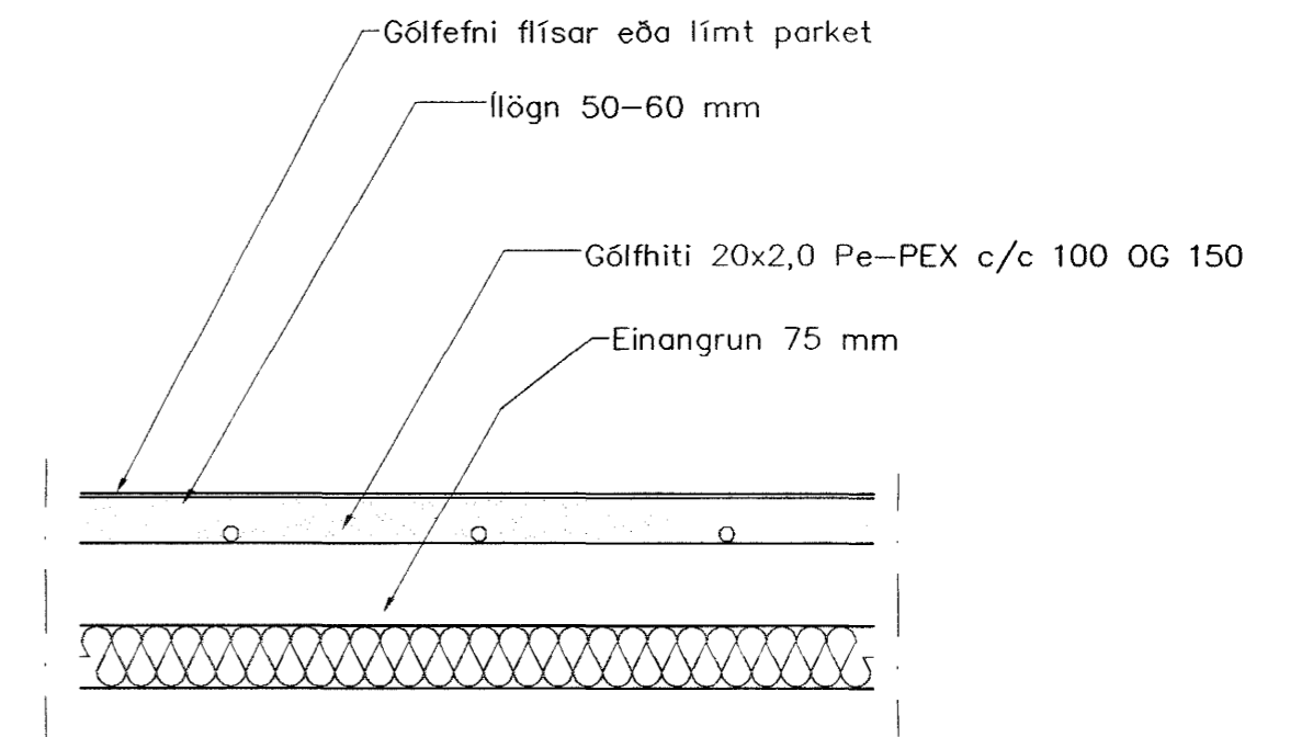
GÓLFHITI SNIÐ, 1:20
