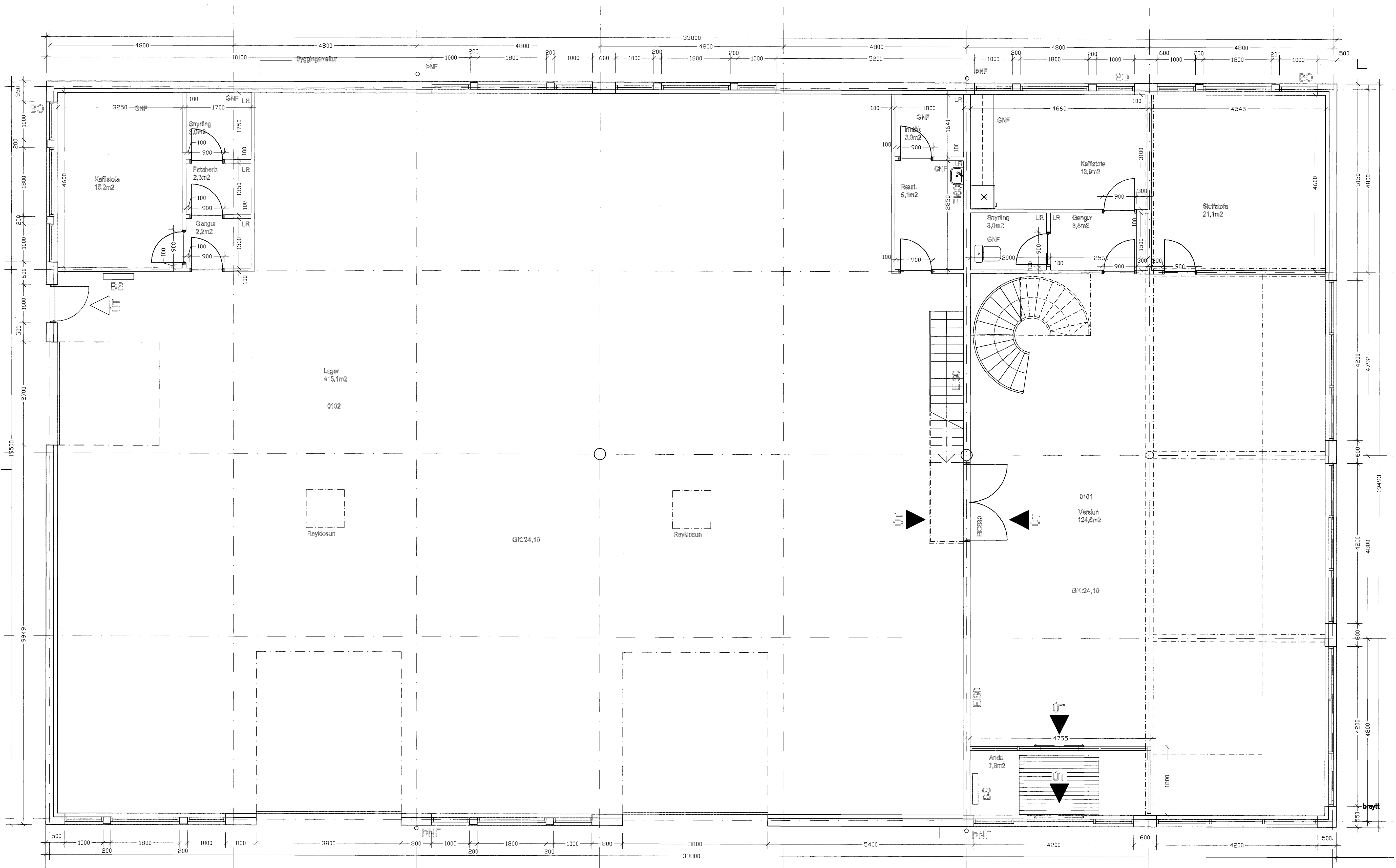
Grunnmynd 1 hæð
