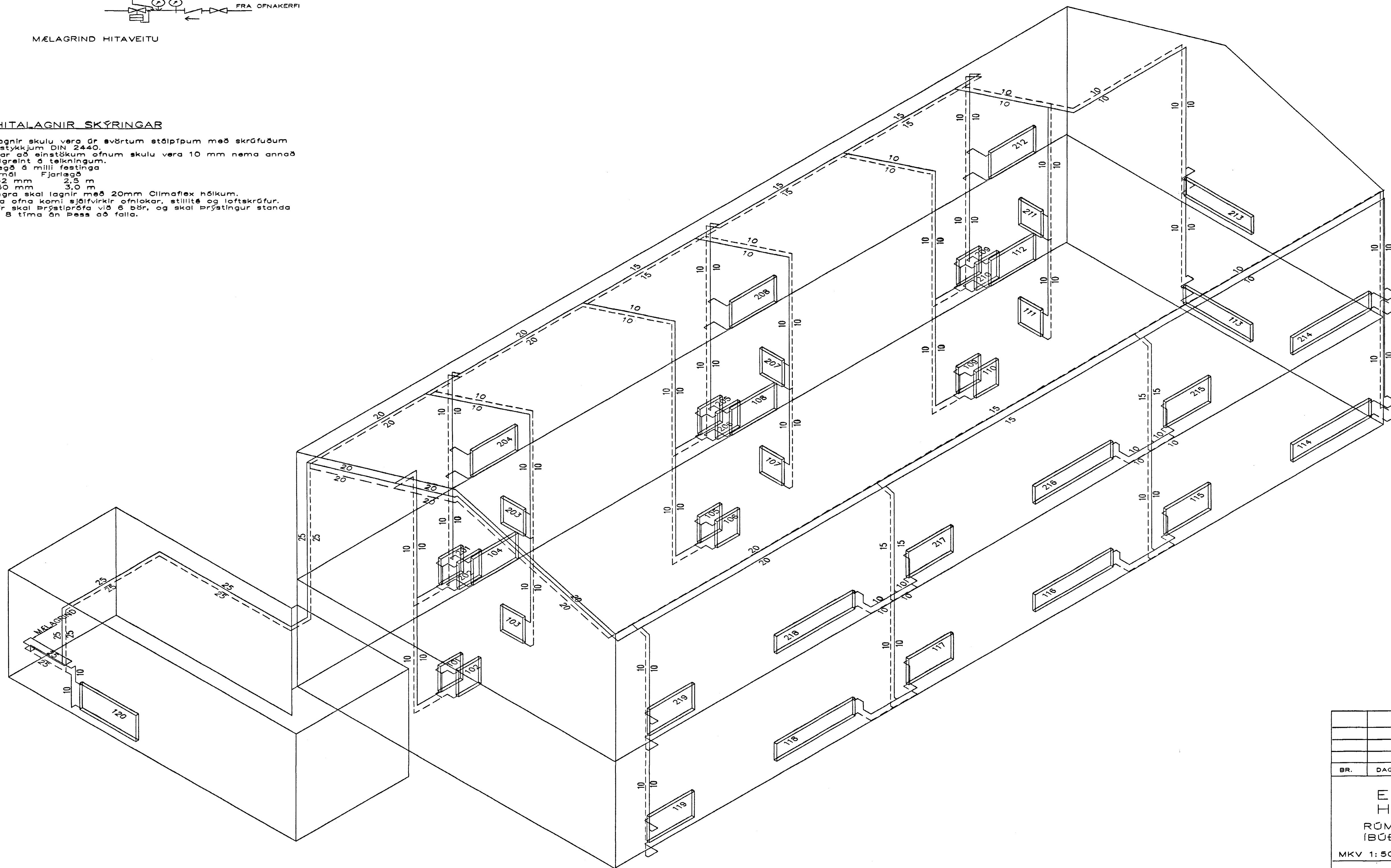
RÚMMYND HITALAGNA 1:50
