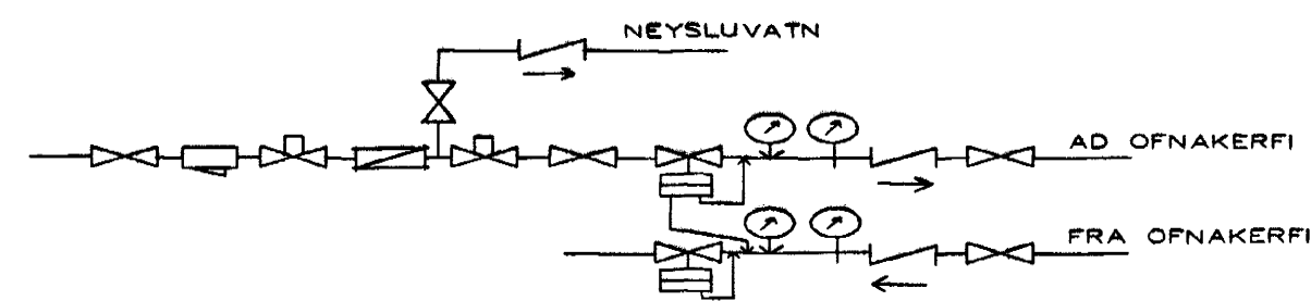
MELAGRIND HITAVEITU
