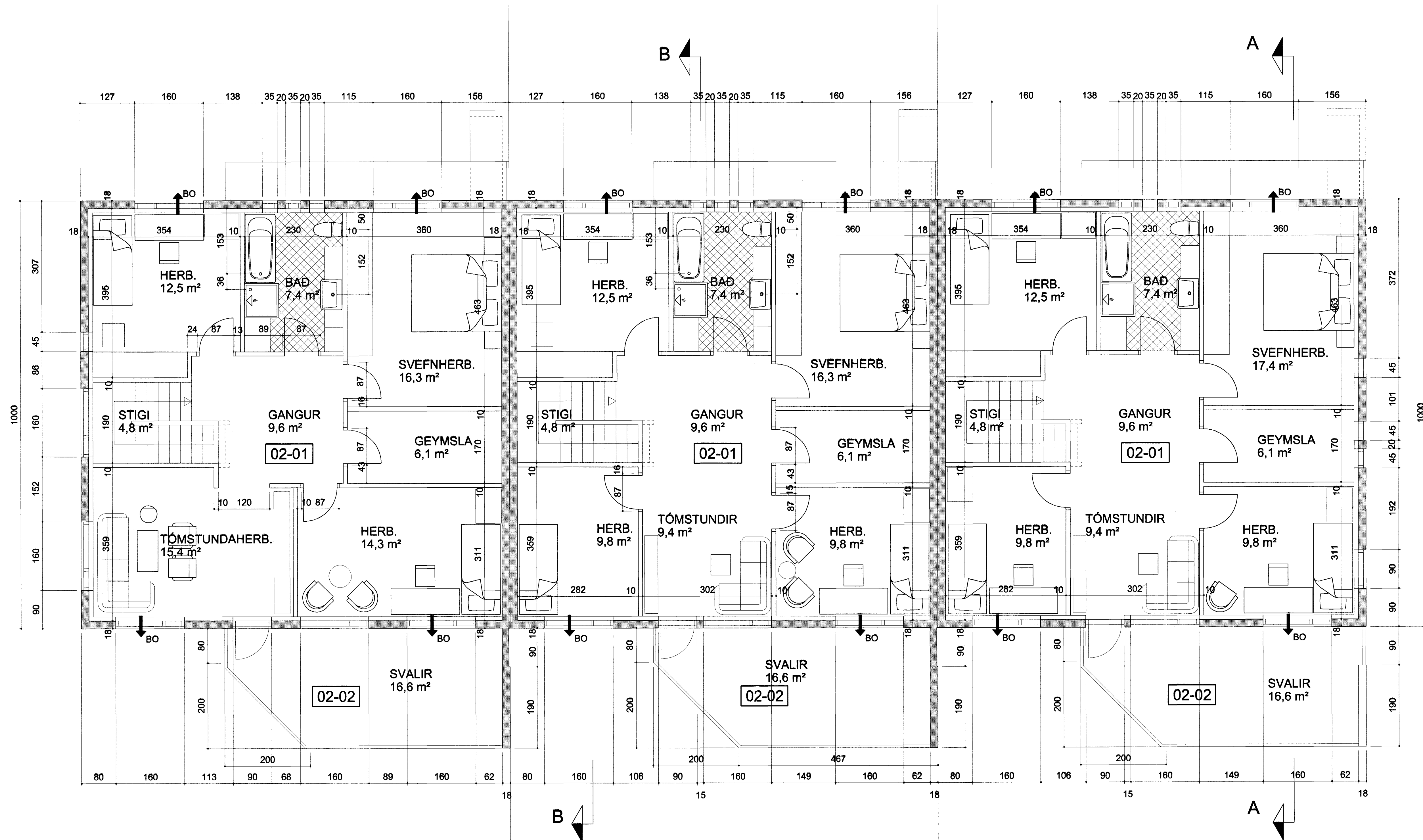
GRUNNMYND 1. HÆÐ 1 : 50
