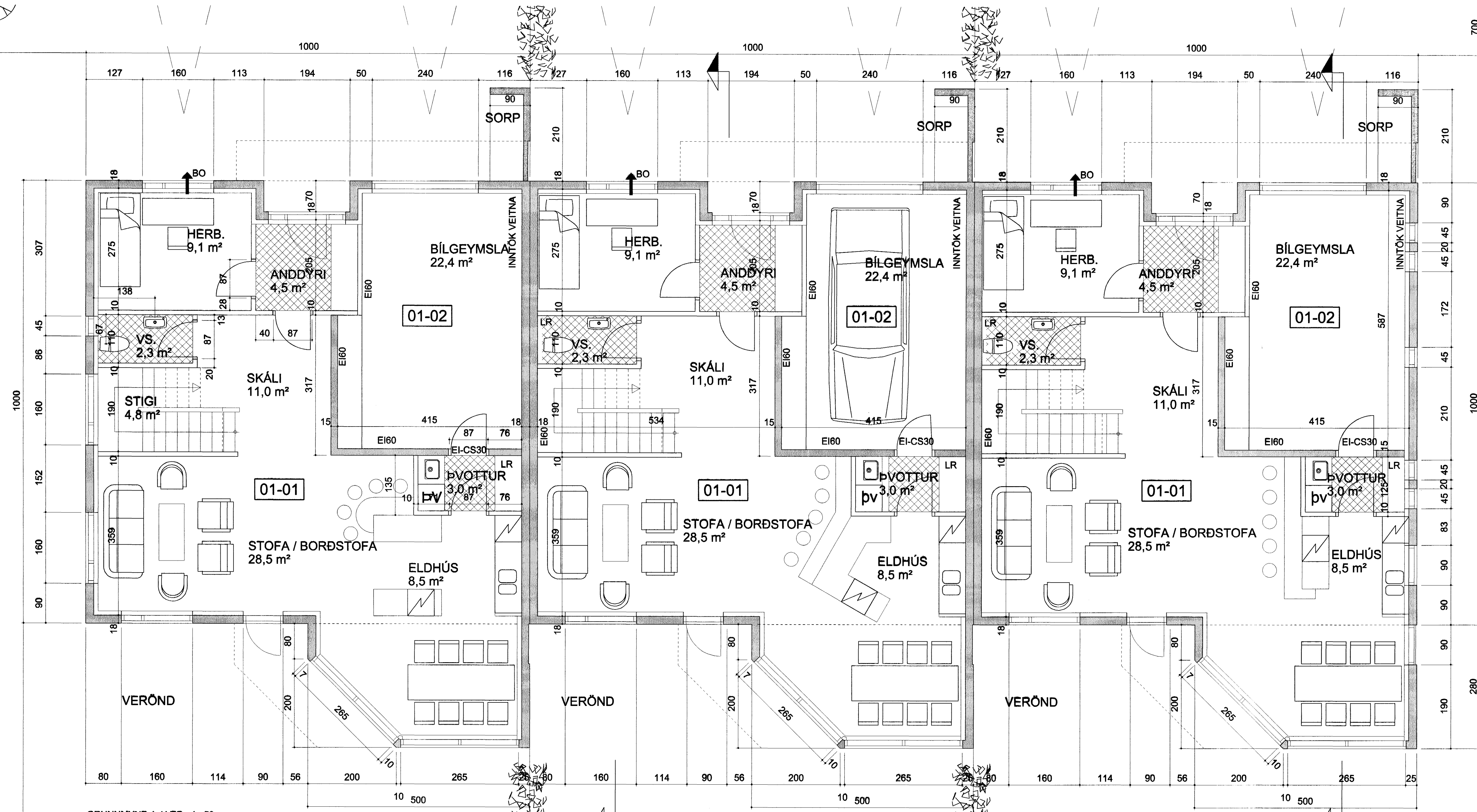
GRUNNMYND 1. HÆÐ 1:50
