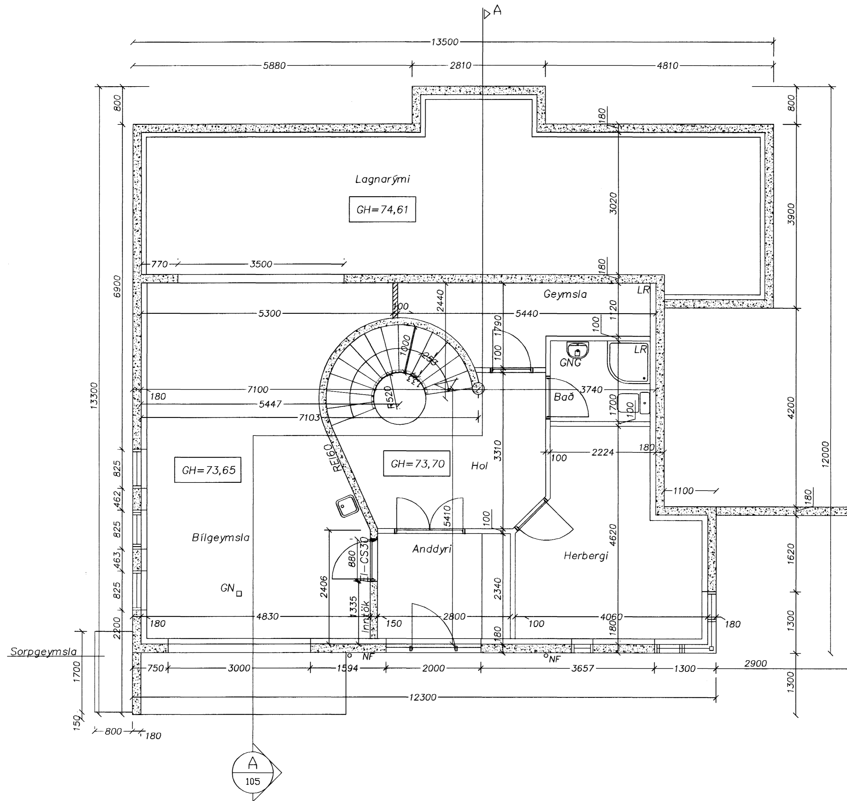
Grunnmynd, neðri hæð Mælikvarði 1:50
