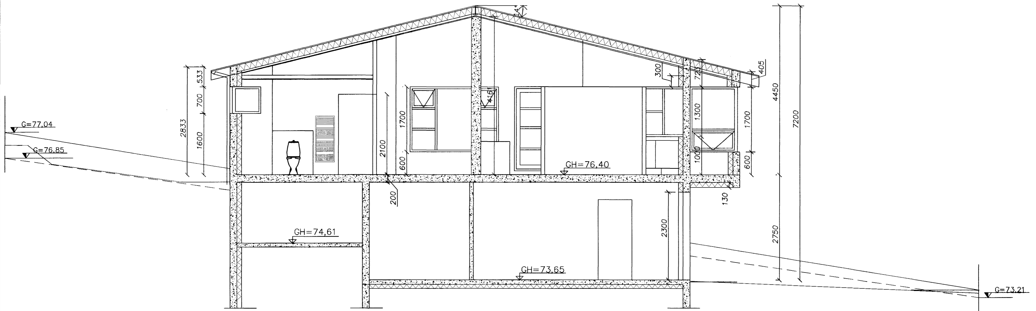
A Snið Málkvarði 1:50
