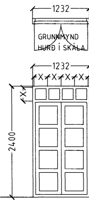
1 STK. SKÁLI. HURÐIR OPNAST ÚT.
