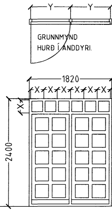
1 STK. ANDDYRI. HURÐ OPNAST VINSTRI ÚT.
