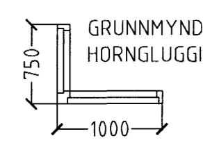
HORNGLUCCI. 1 STK. SKÁLI.
