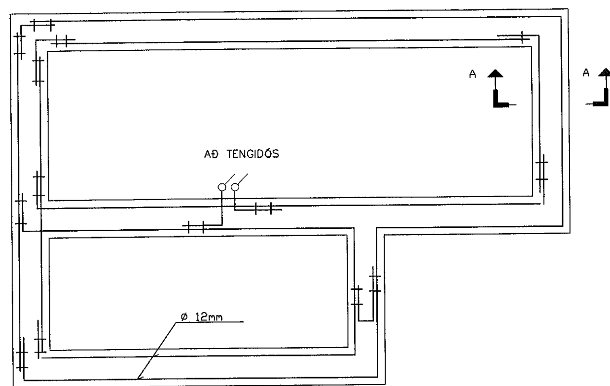
GRUNNMYND SÖKKULVEGGJA
