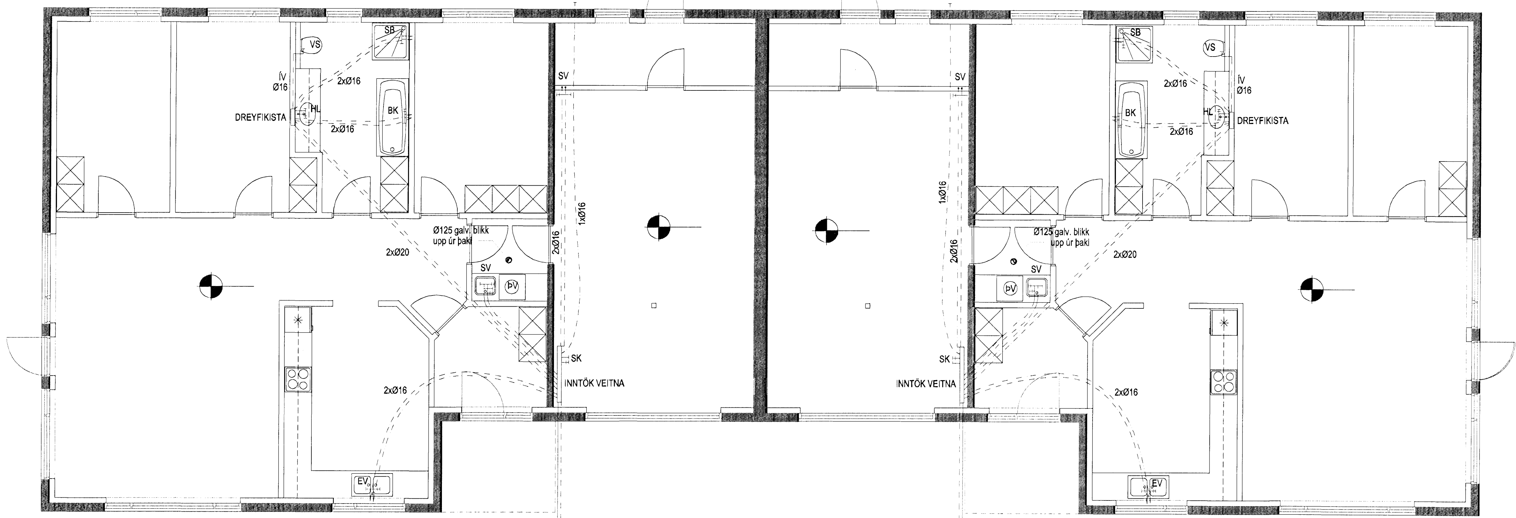
NEYSLUVATNSLAGNIR, GRUNNMÝND MKV. 1:50
