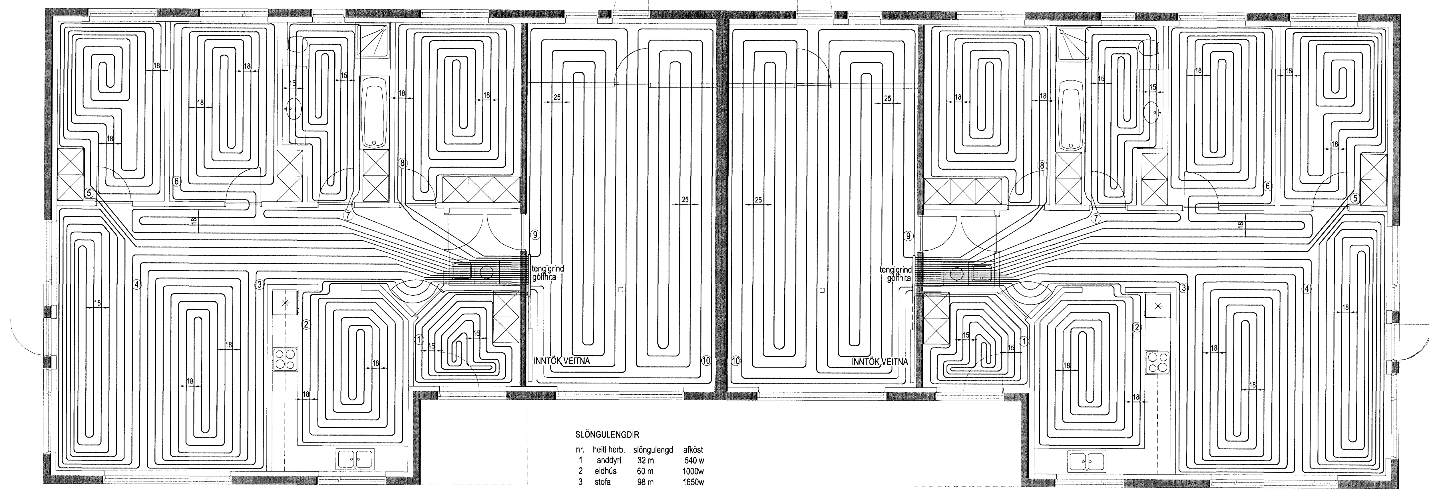
GÓLFHITALAGNIR, GRUNNMÝND MKV. 1:50
