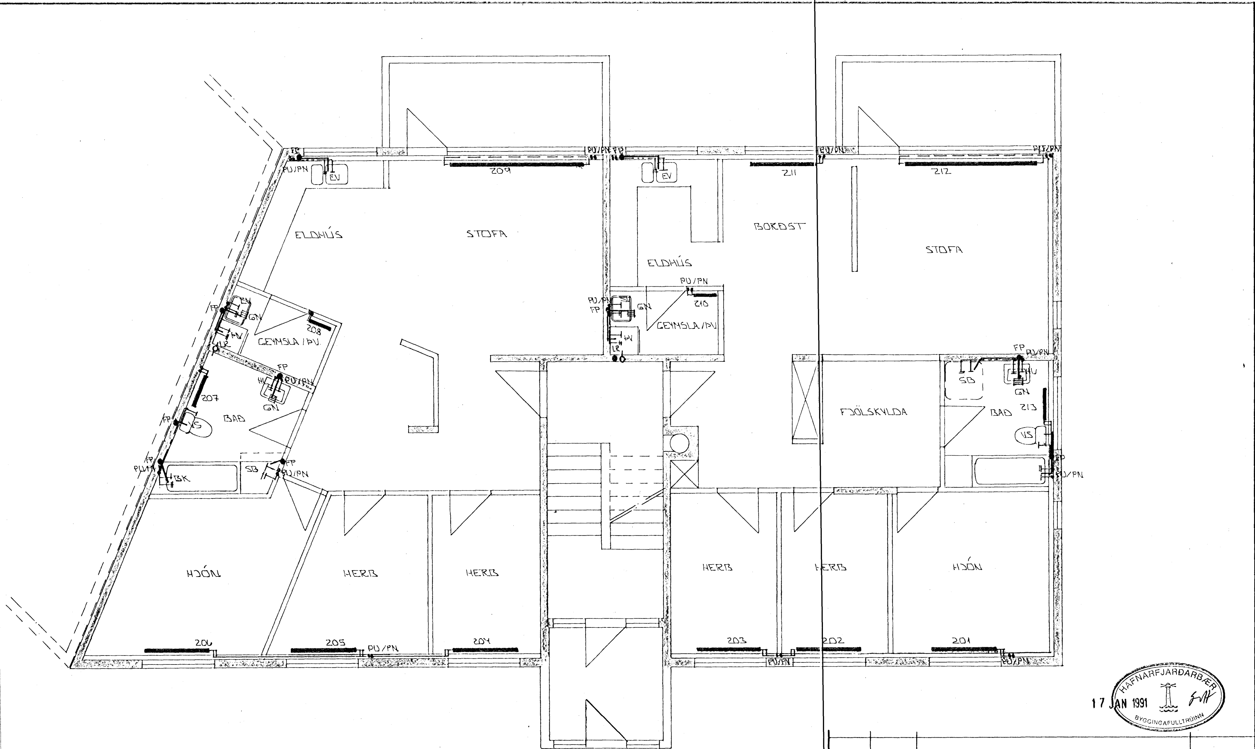
GRUNNMÝND 2. HÆÐAR 1:50
