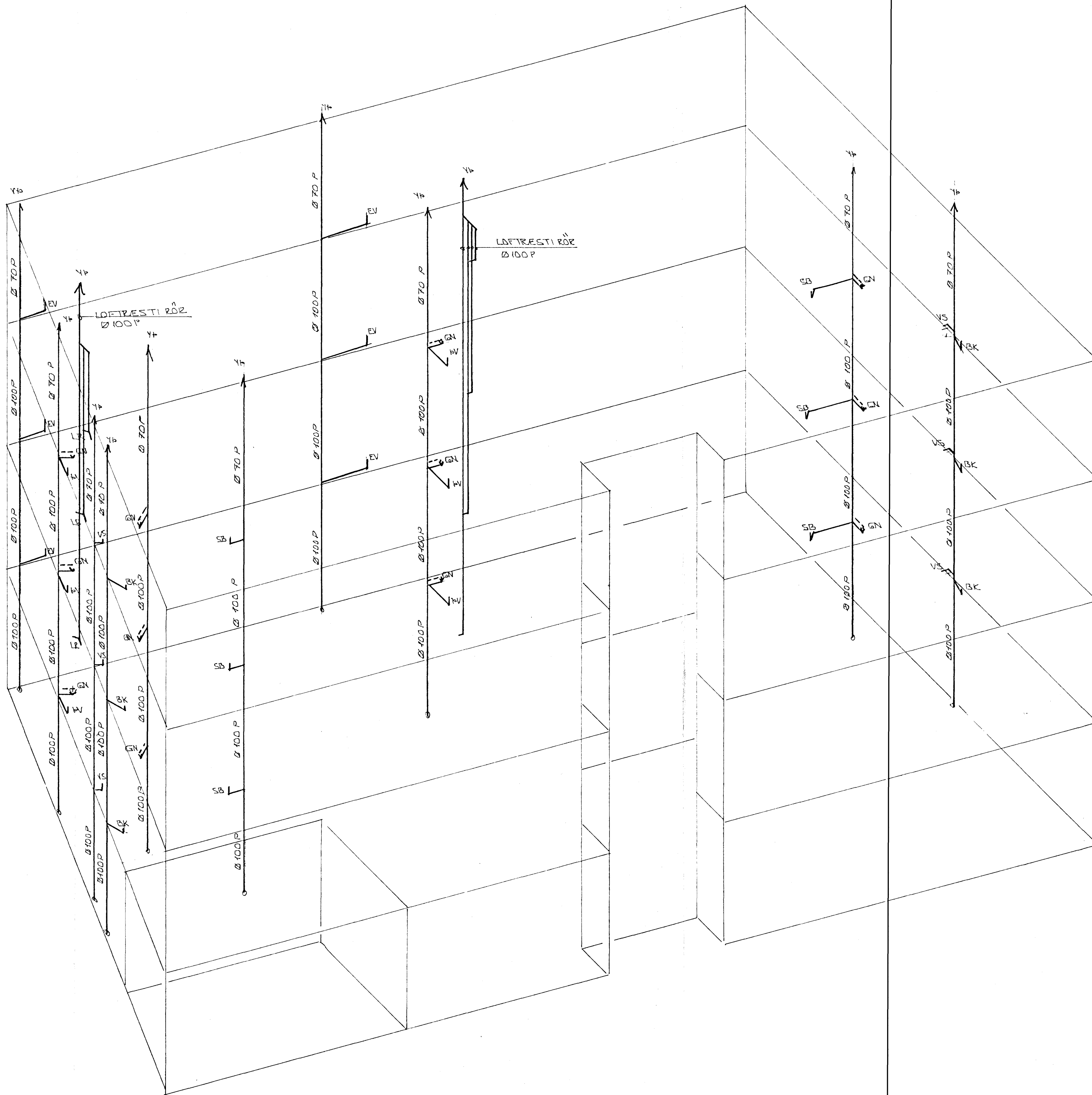
RÚMMYND FRÆNNSLIS- OG LOFTRESTILAGNA 1:50
