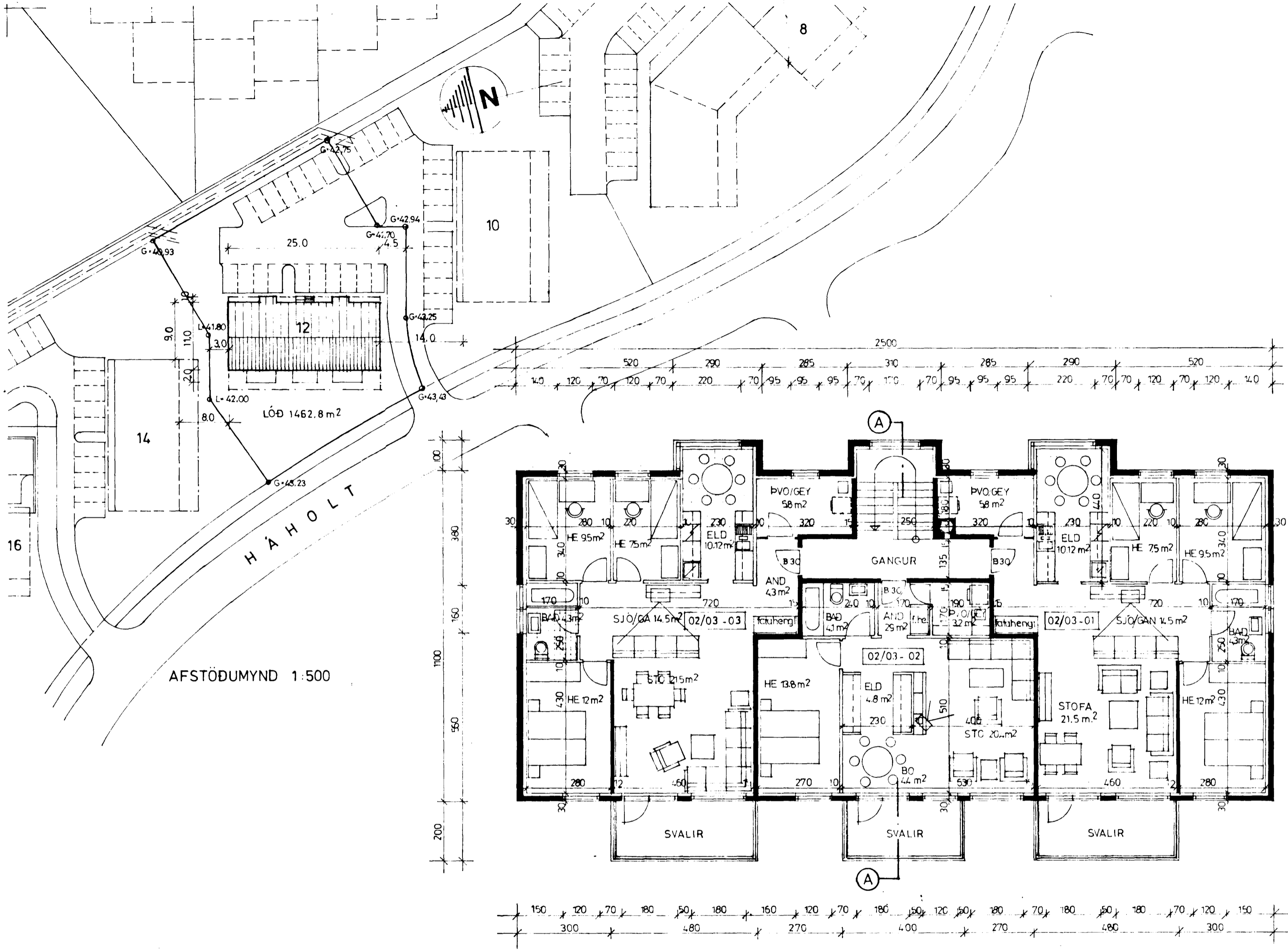
GRUNNMYND 02 & 03 1:100
