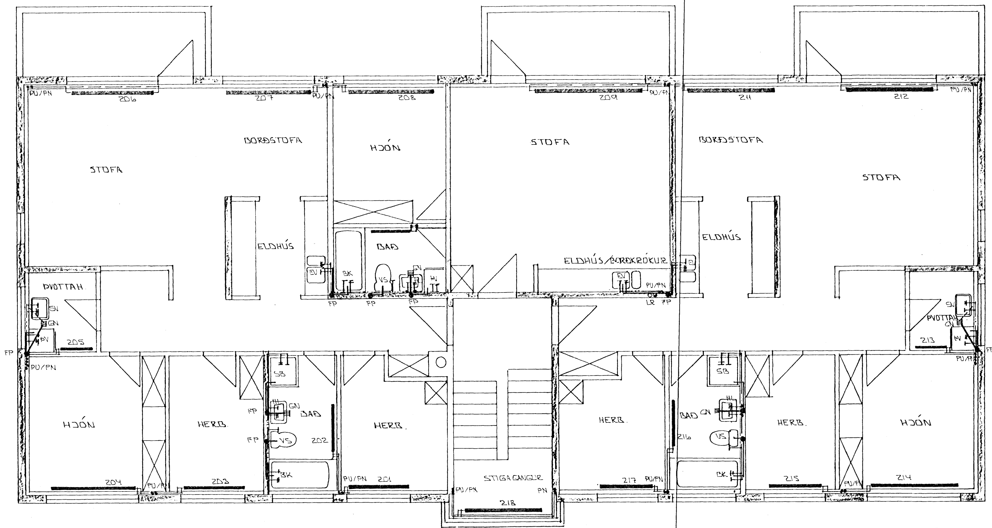
GRUNNMÝND 2. HÆÐ 1:50
