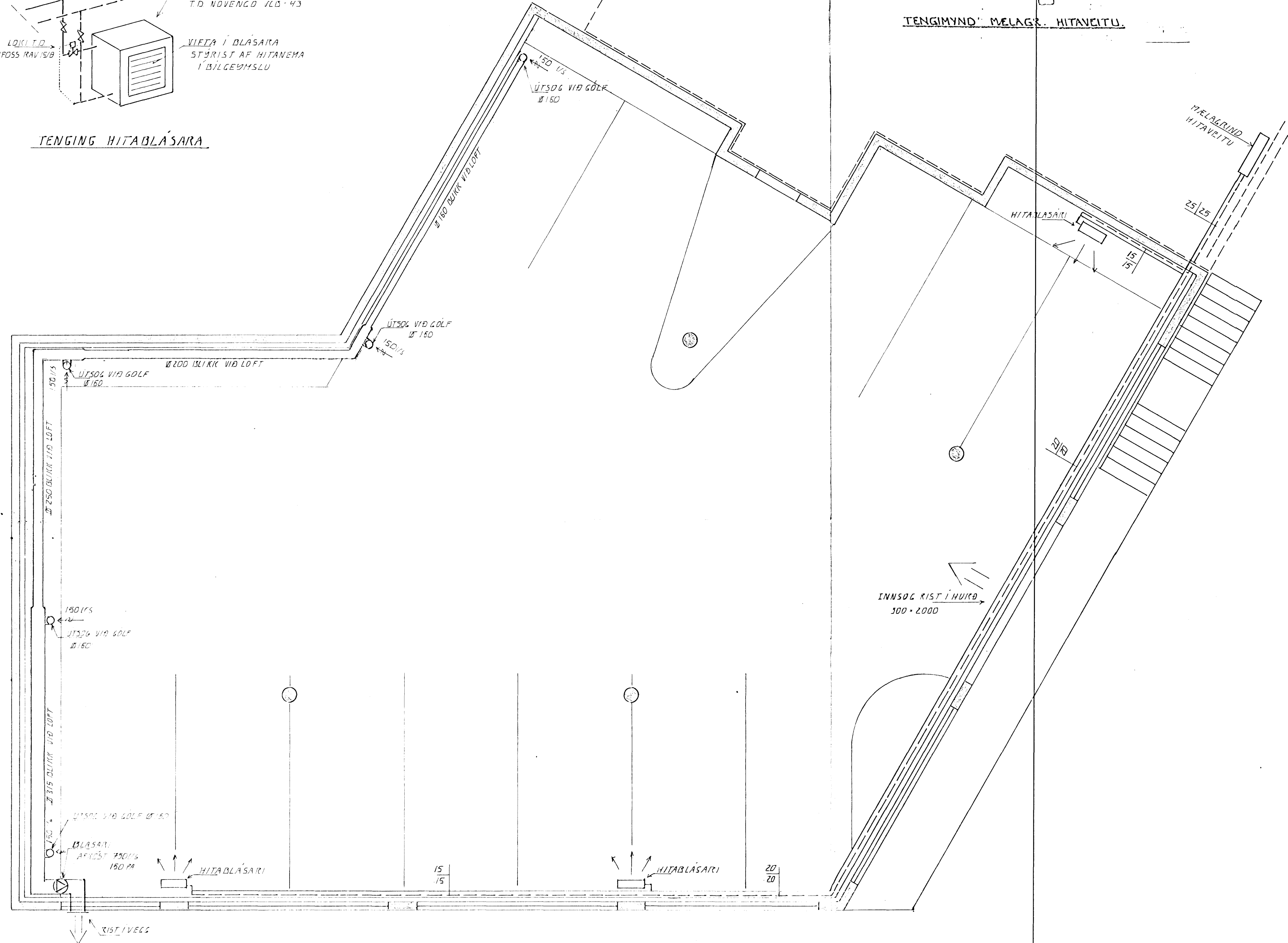
BÍLGEYMSLA GRUNNMÝND 1:50
