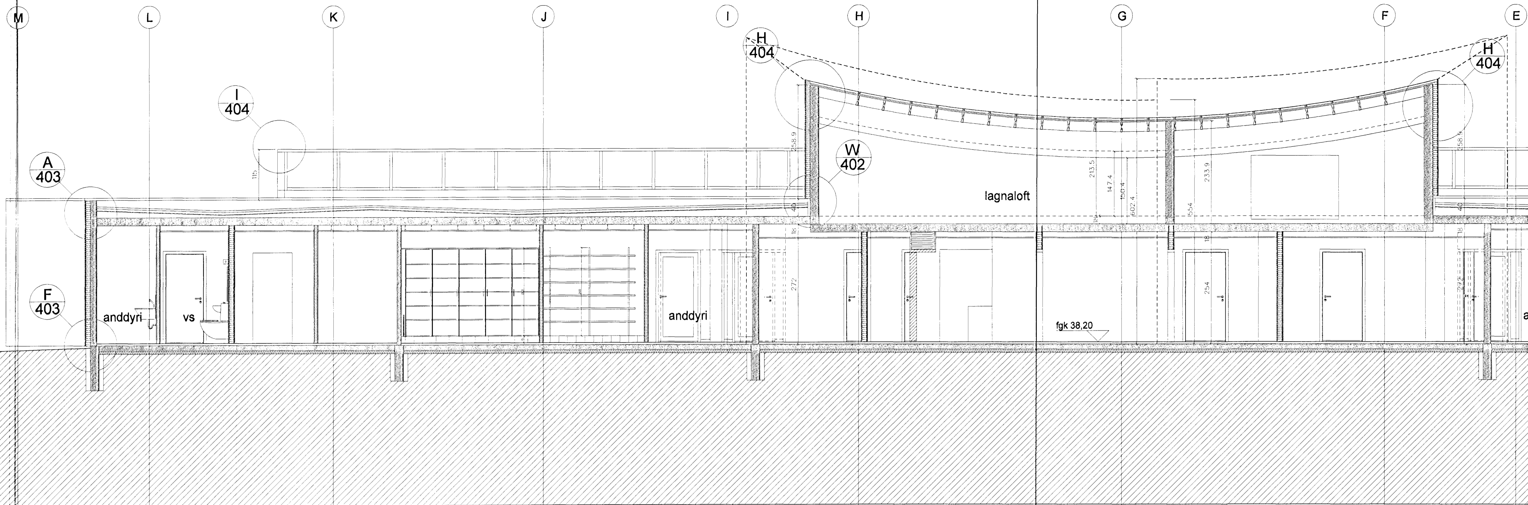
langskurður D - D austurhluti
