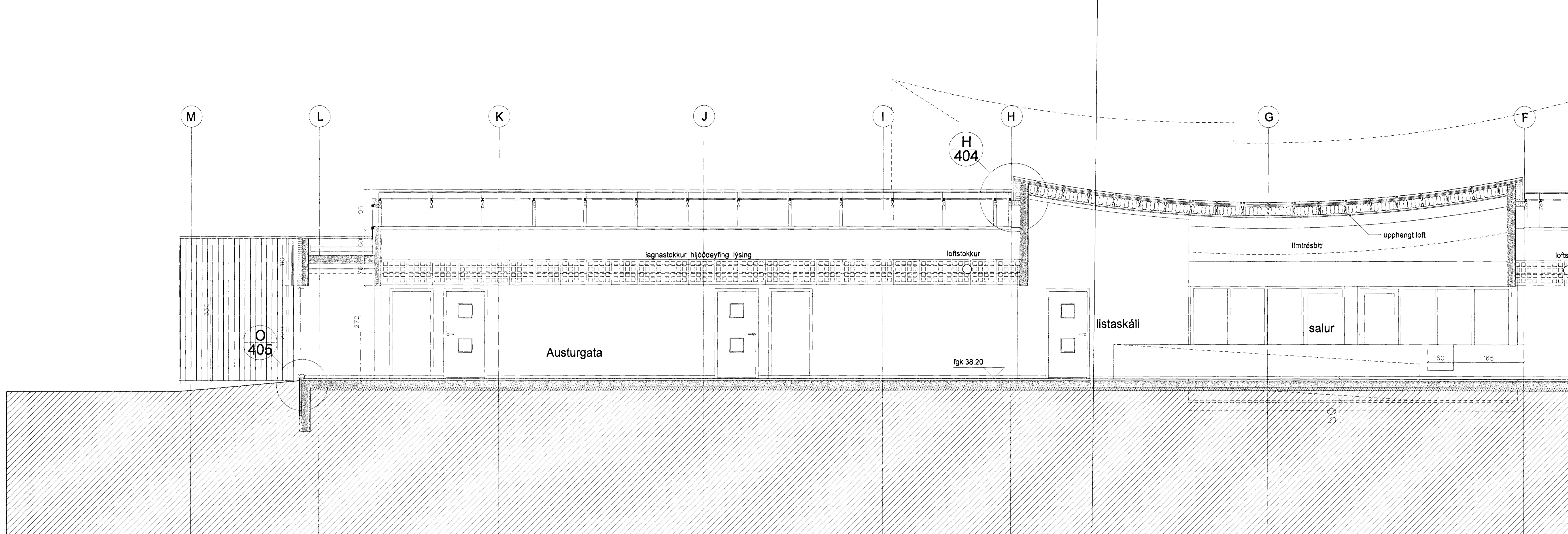
langskurður G - G vesturhluti
