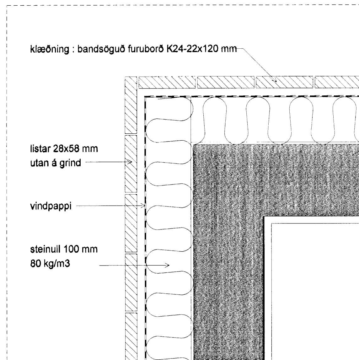
lárétt deili 402 L á úthorni
