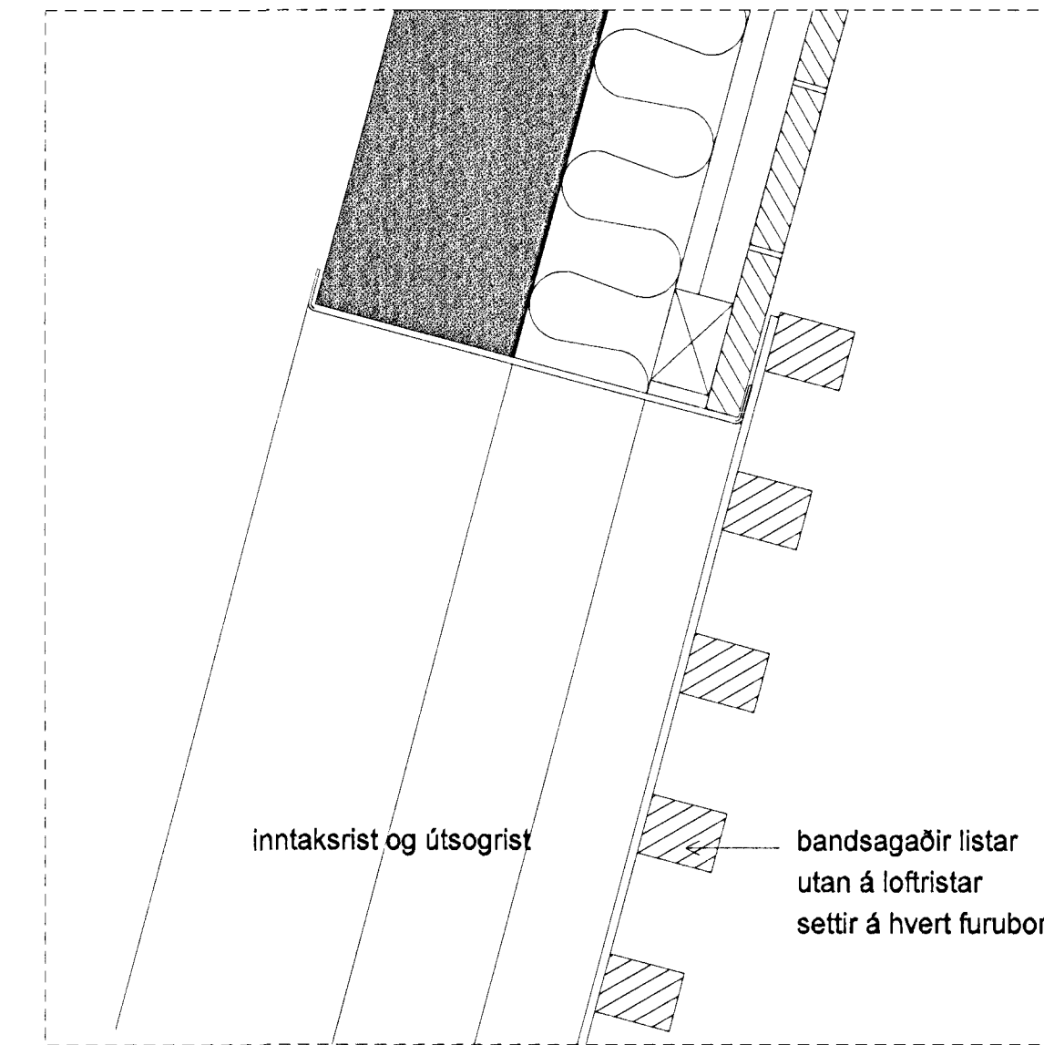
deili O-402 yfir inntaksrist
