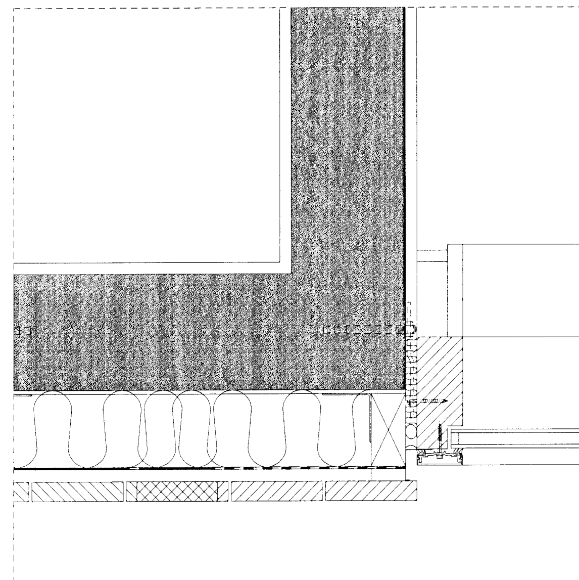
lárétt deili 402 R innhorn við glugga
