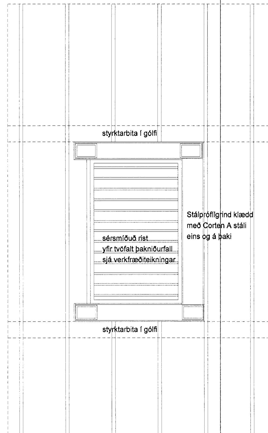
lárétt deili T-402 í þakniðurfall
