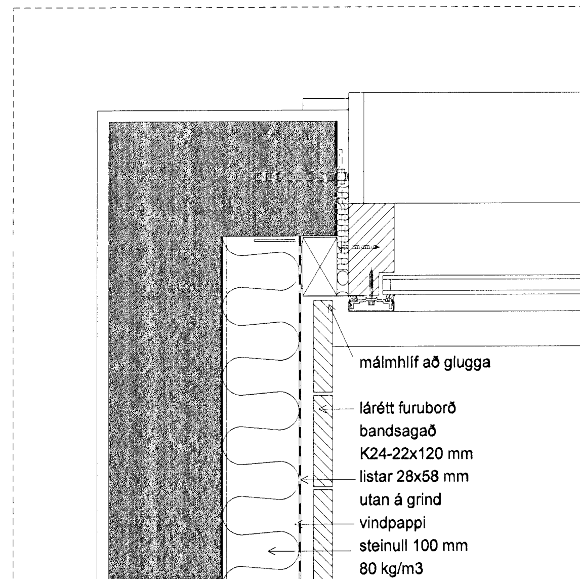
lárétt deili P-402 innhorn við glugga
