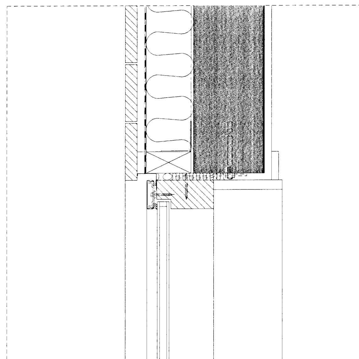
lárétt deili 402 M við glugga
