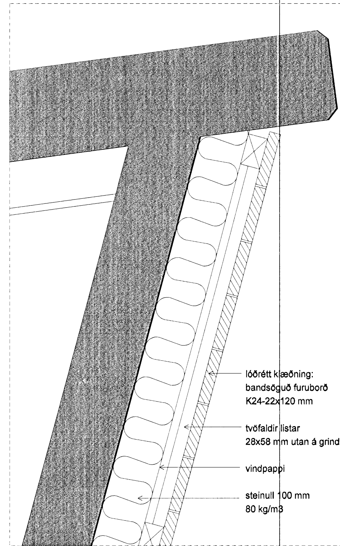
deili P-402 ofan við glugga á norðurhlíð
