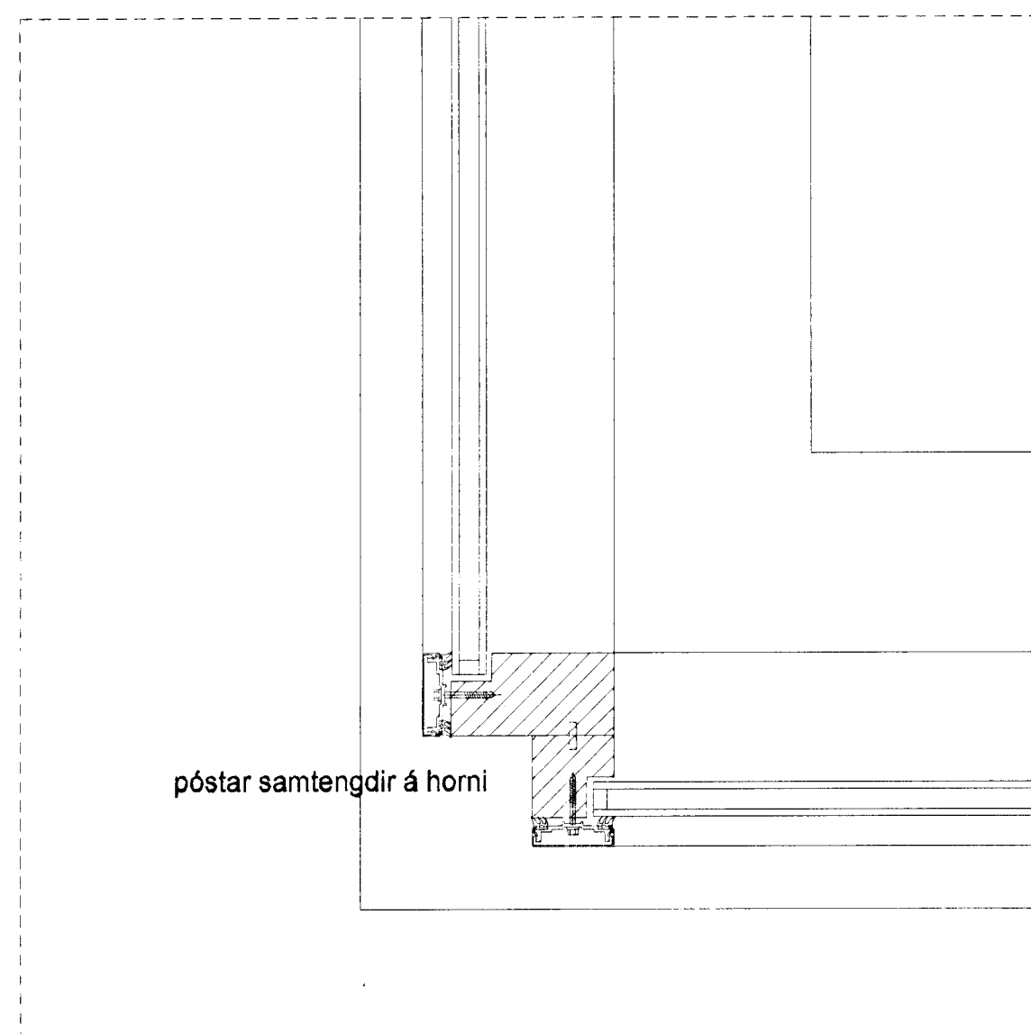
lárétt deili 402 N úthorn glugga
