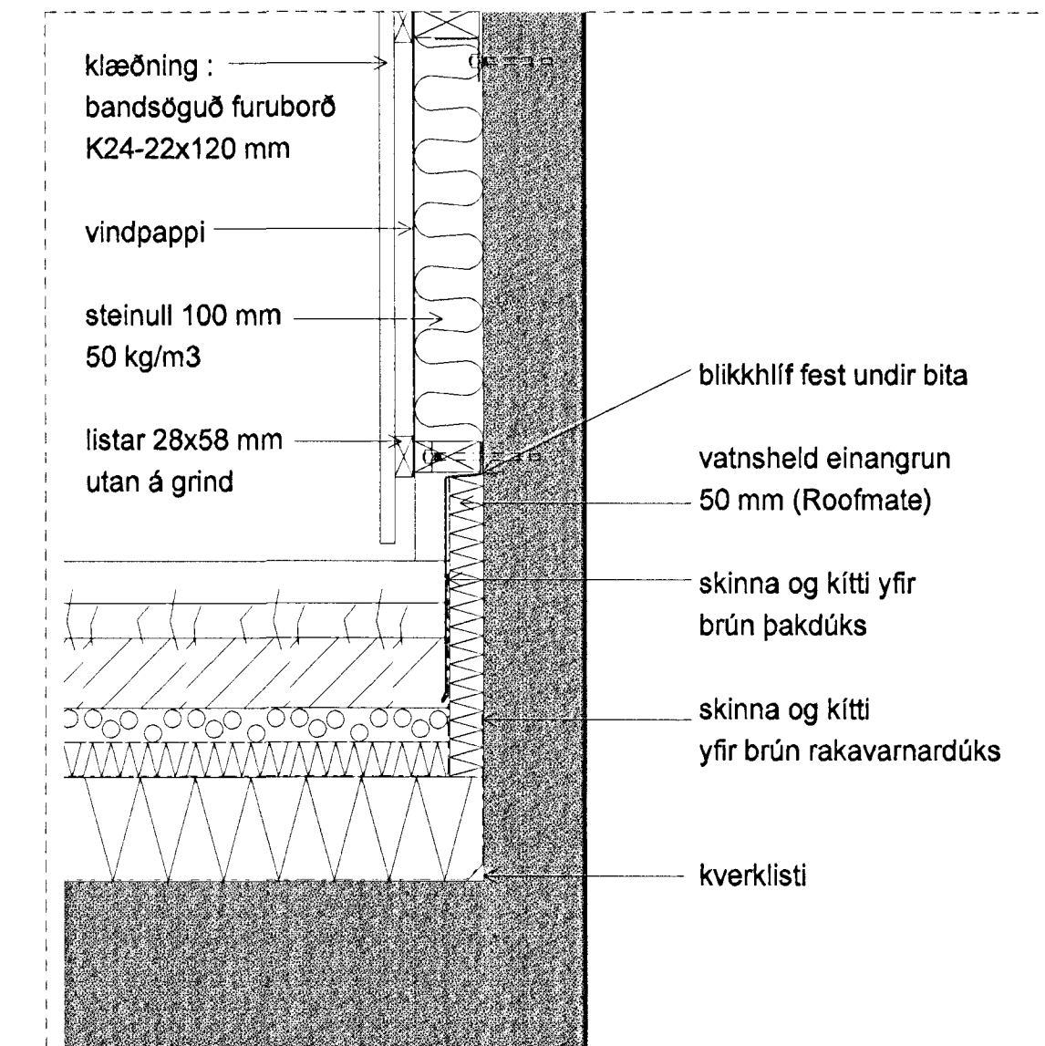
lóðrétt deili W-402
