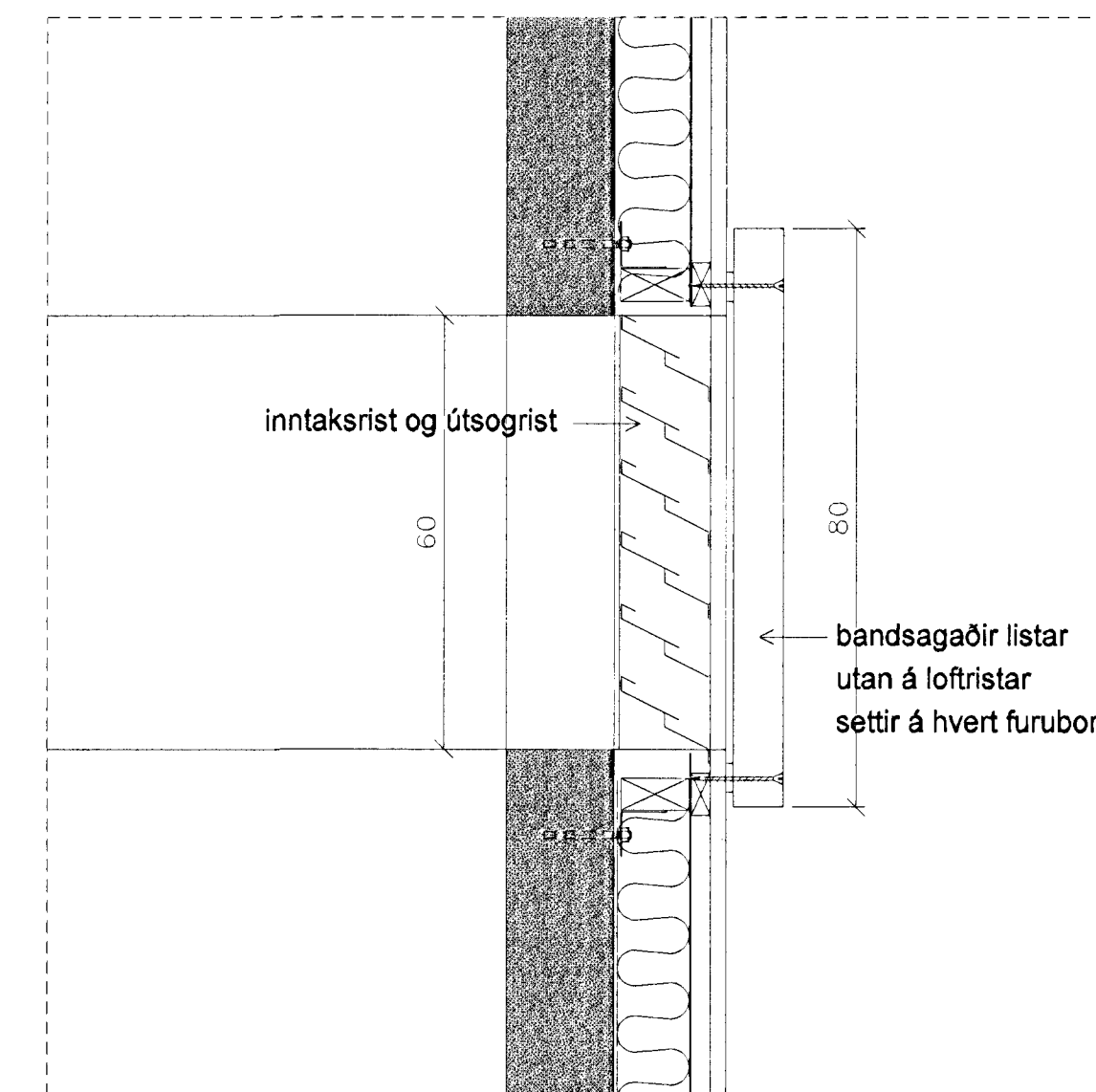
lóðrétt deili V-402
