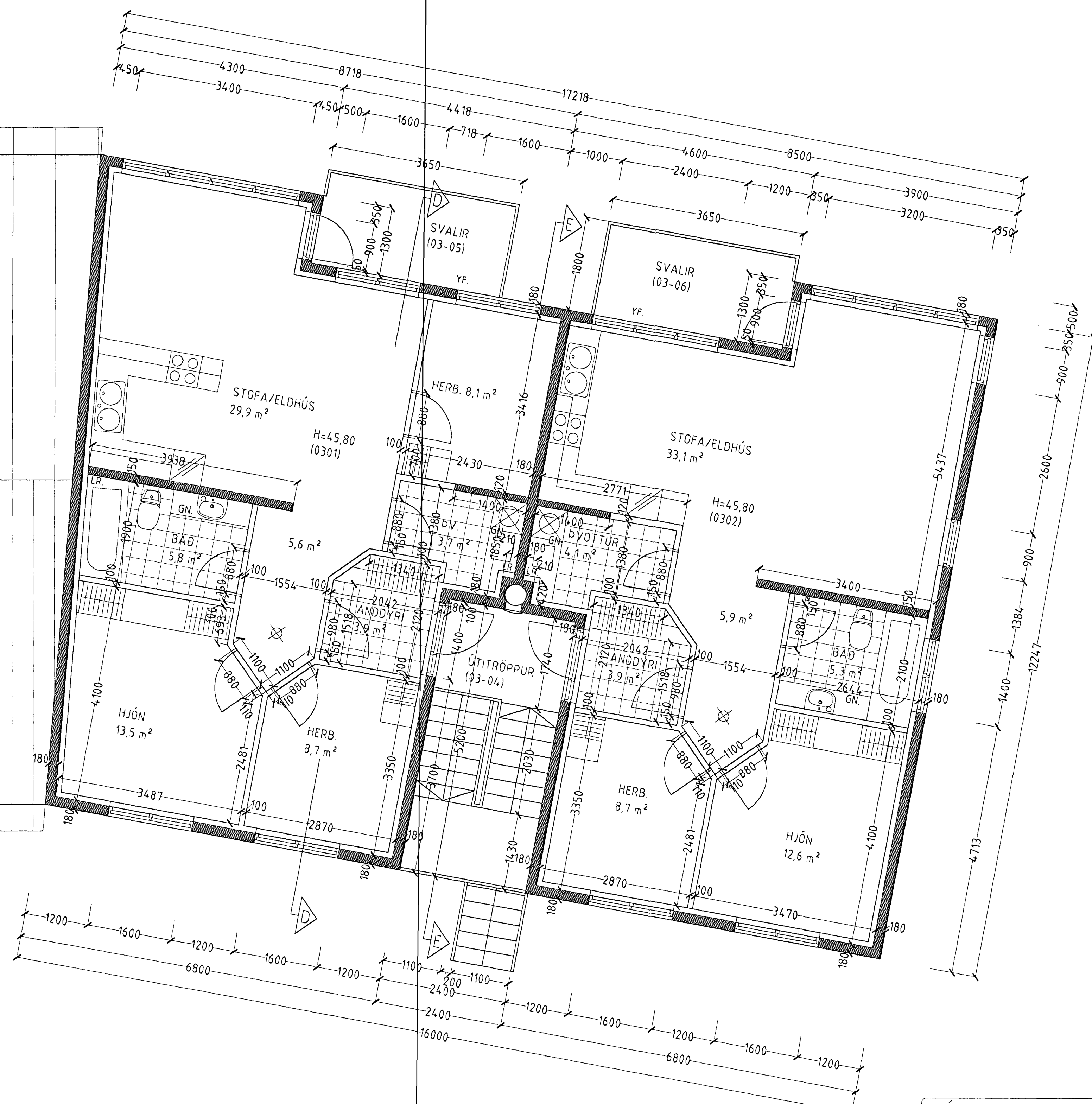
GRUNNMYND 3. HÆÐ MKV. 1:50.
