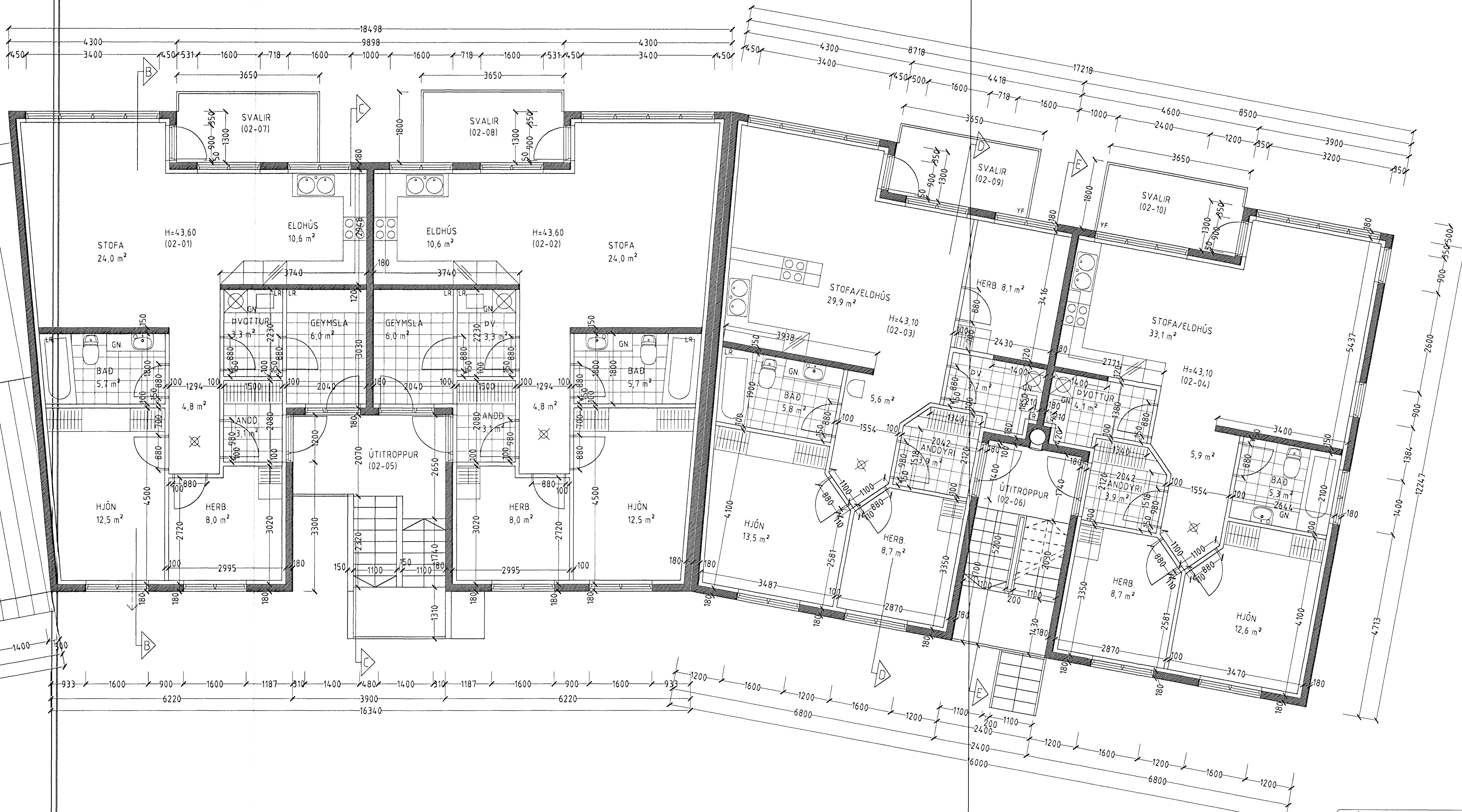
GRUNNMYND 2. HÆÐ MKV. 1:150.
