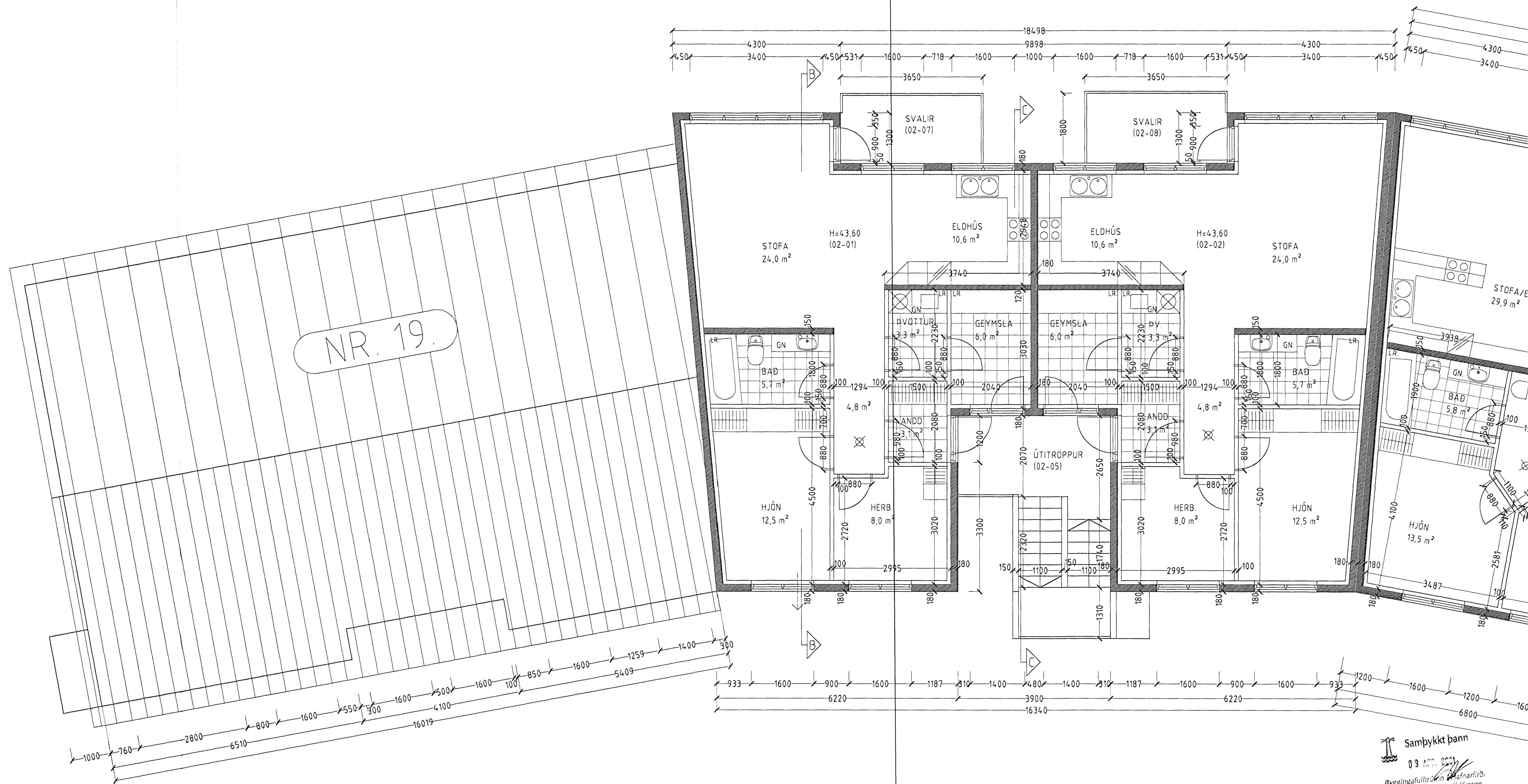
GRUNNMYND 2. HÆÐ MKV. 1:150.
