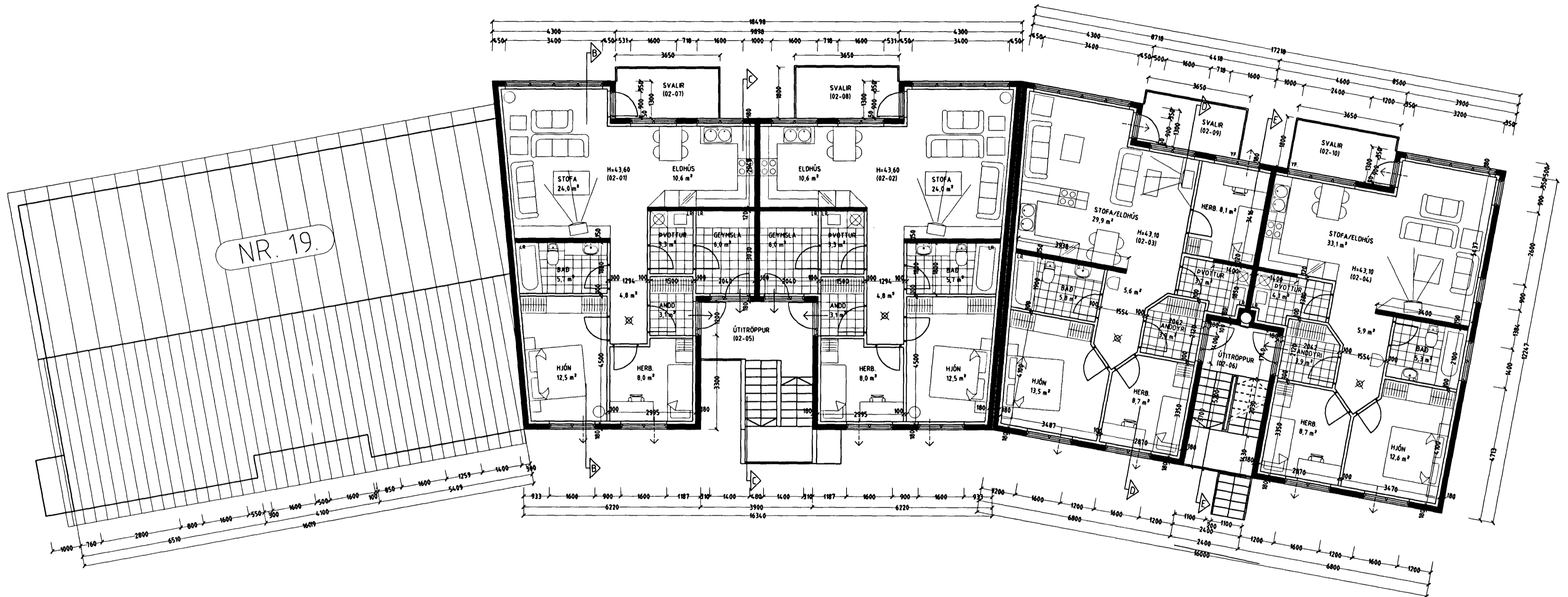
GRUNNMYND 2 HÆÐ MKV. 1:100.
