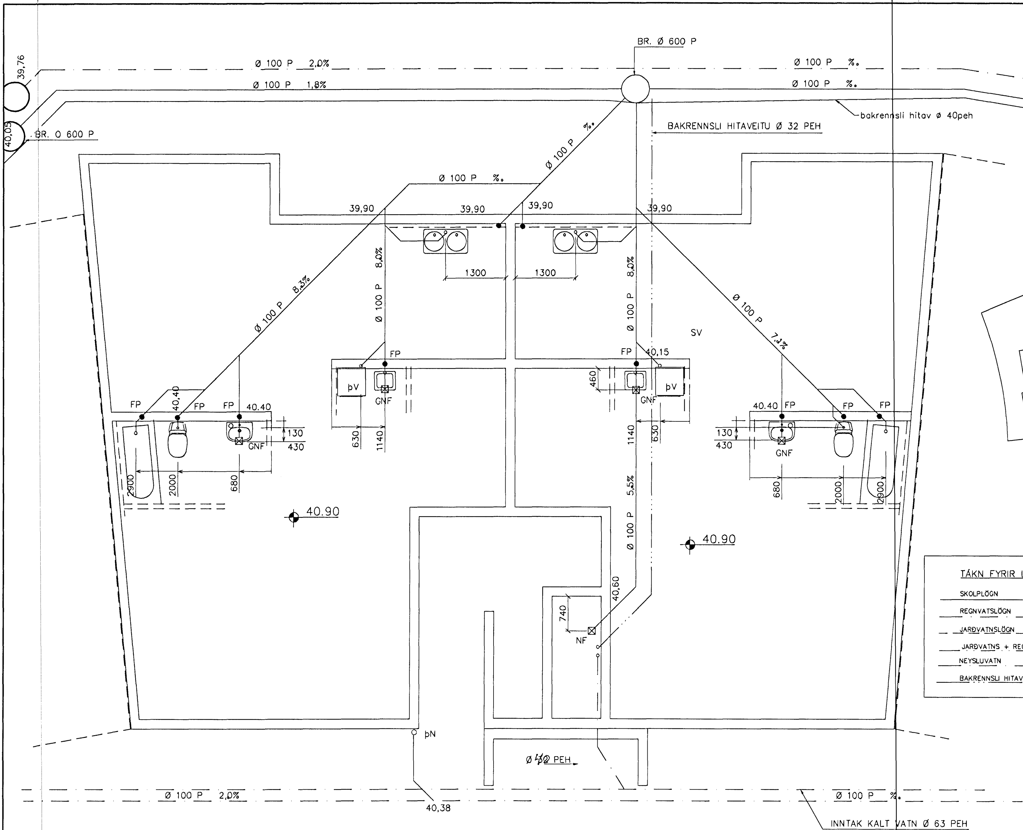
GRUNNMYND 1:50
